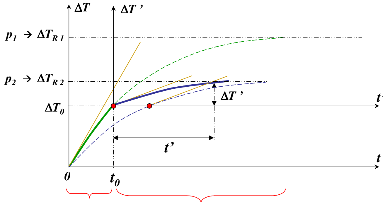
EVOLUÇÃO DA SOBRELEVAÇÃO DE TEMPERATURA COM VARIAÇÃO DE PERDAS
