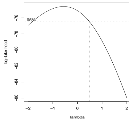
Figura 4.8: Gráfico do perfil de verossimilhança para a transformação de Box-Cox .
