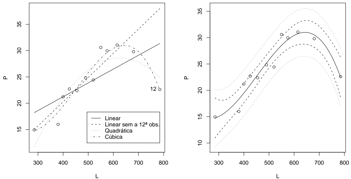
Figura 4.11: Gráfico de dispersão e modelos ajustados e gráfico de dispersão com intervalos de 95% de confiança para a resposta média E(P) (---) e para a resposta predita \hat{P} (···), supondo o modelo de regressão cúbica.
