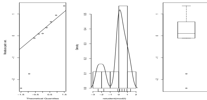
Figura 4.3: Gráfico normal de probabilidades, histograma e boxplot dos resíduos estudentizados externamente (rse).
