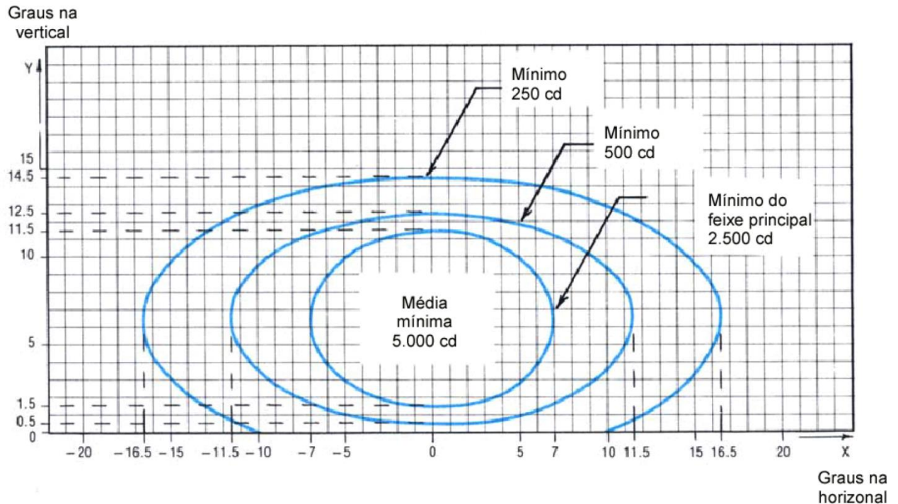
Figura AB-2. Diagrama de isocandela para as luzes da fileira lateral de aproximação (luz vermelha)
