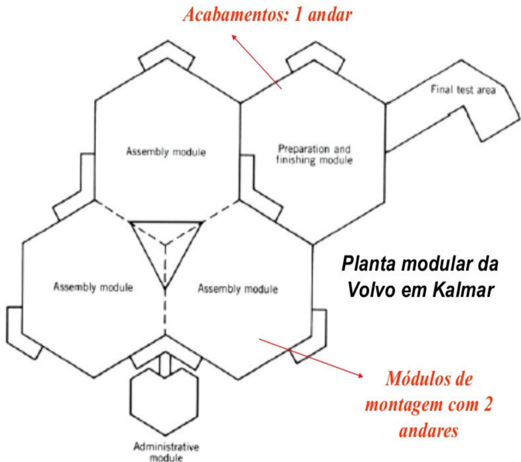
Figura 3 – Planta modular da Volvo em Kalmar.
