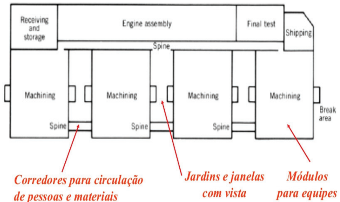
Figura 2 – Visão da área de fabricação de motores (Skovderken).
