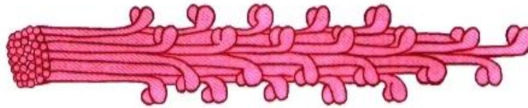
Fig. 22.3 Esquema mostrando a posição relativa de moléculas de miosina compondo parte de um filamento grosso (a extremidade do lado direito, na banda A da Fig. 22.1).
