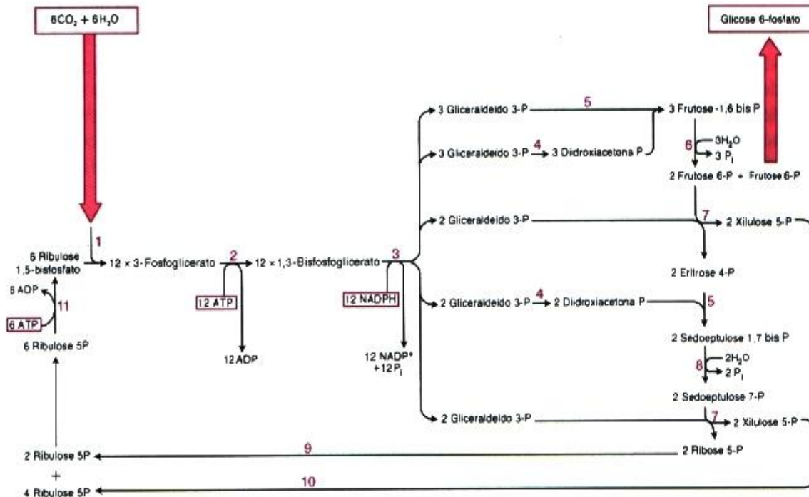
Fig. 15.10 Ciclo de Calvin. O esquema mostra a síntese de uma molécula de glicose 6-fosfato a partir de 6 moléculas de CO_2 e 6 moléculas de H_2O . O esquema inicia-se com 6 moléculas de ribulose 1,5-bisfosfato que são regeneradas no fim do ciclo. Os números nas setas referem-se às enzimas: rubisco (1), fosfoglicerato quinase (2), gliceraldeído 3-fosfato desidrogenase (3), triose fosfato isomerase (4), aldolase (5), frutose 1,6-bisfosfatase (6), transcetolase (7), sedoheptulose 1,7-bisfosfatase (8), ribose fosfato isomerase (9), fosfopento epimerase (10) e ribulose 5-fosfato quinase (11).
