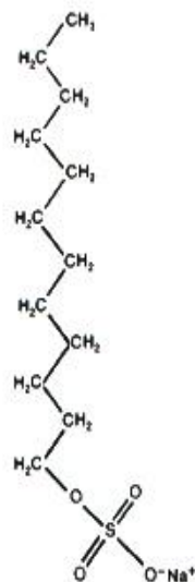
Fig. 2.16 O detergente dodecil sulfato de sódio (SDS).
