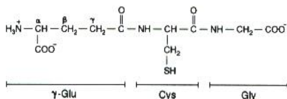
Fig. 12.3 Estrutura da glutaciona, um tripeptídio formado por glutamato, cisteína e glicina; a ligação peptídica entre Glu e Cys é exótica, porque envolve a \gamma -carboxila do glutamato.
