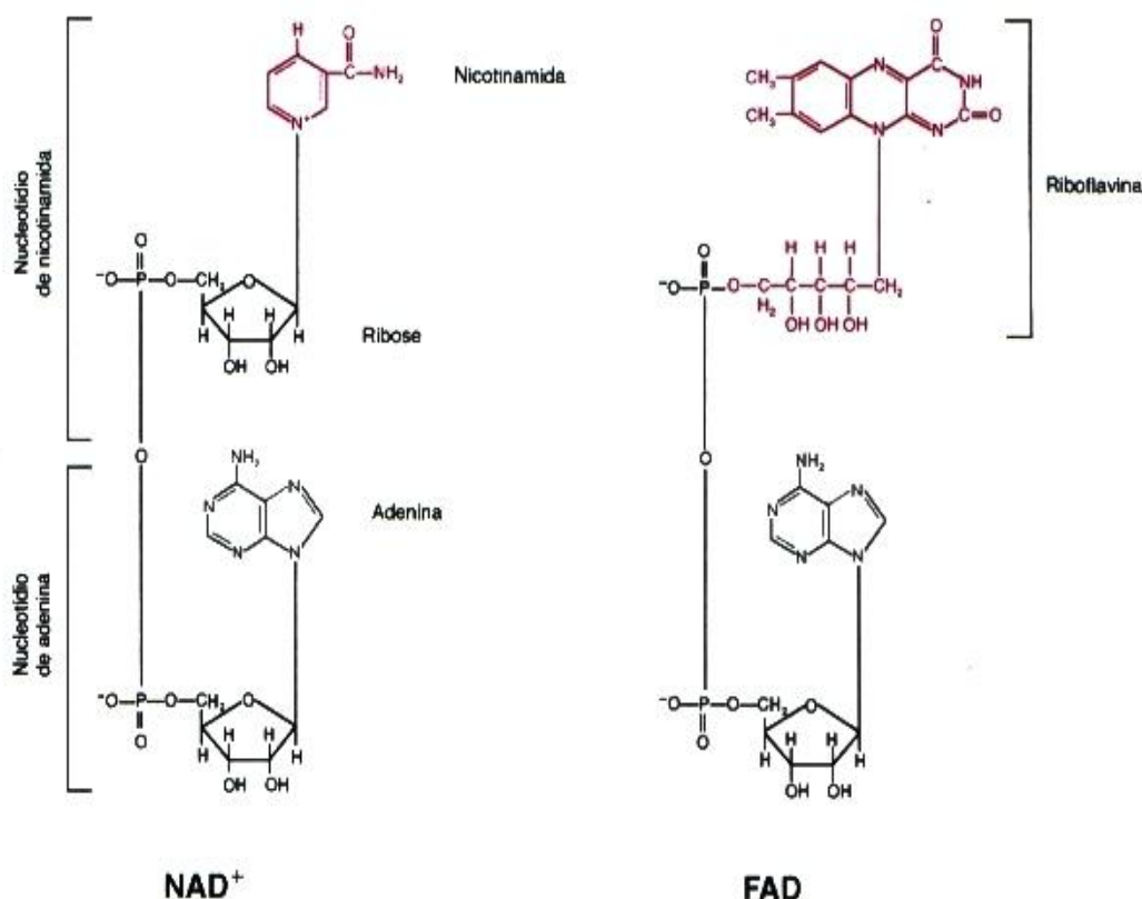
Fig. 9.2 Estrutura das formas oxidadas da nicotinamida adenina dinucleotídio ( NAD^+ ) e da flavina adenina dinucleotídio ( FAD ). Cada nucleotídio é formado por uma base nitrogenada, uma ribose (ou o poliálcool ribitol) e um grupo fosfato. As vitaminas componentes das coenzimas estão destacadas em vermelho.
