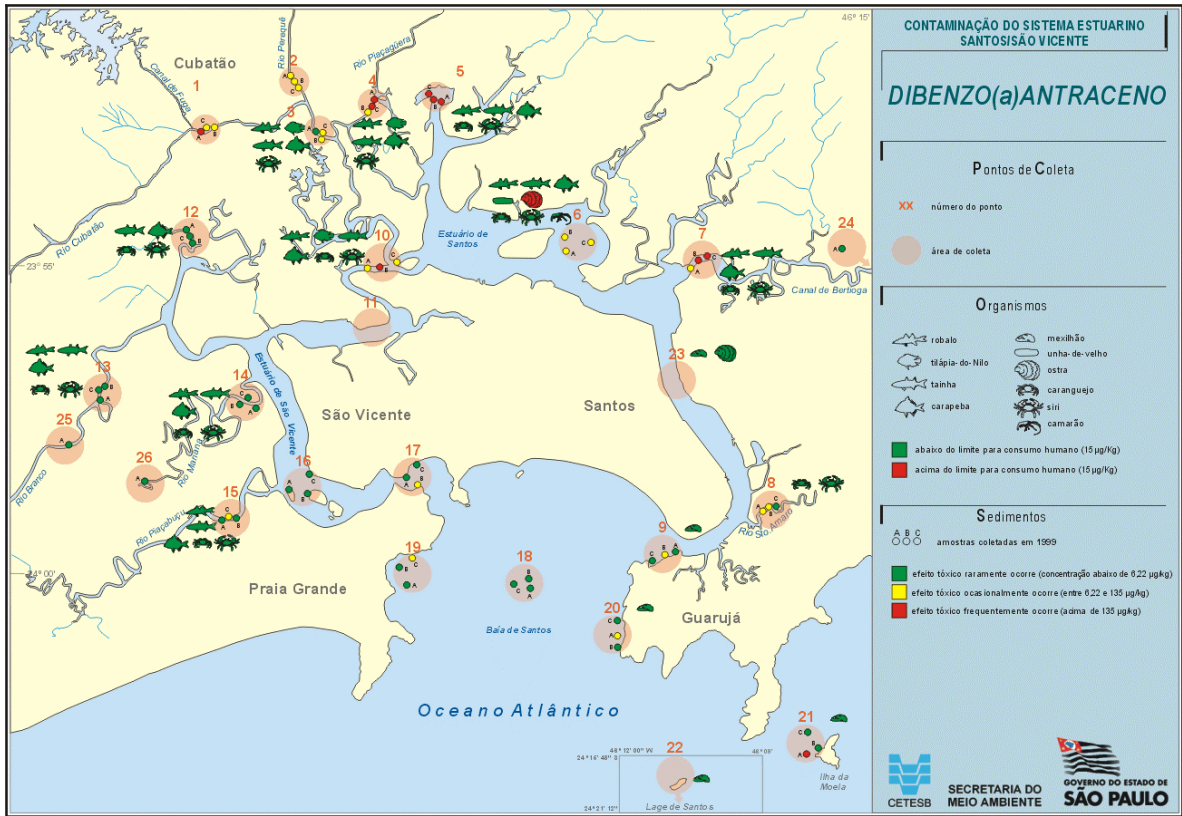
Figura 36- Mapa da contaminação por Dibenzo (a) Antraceno na Baixada Santista em 1999.
