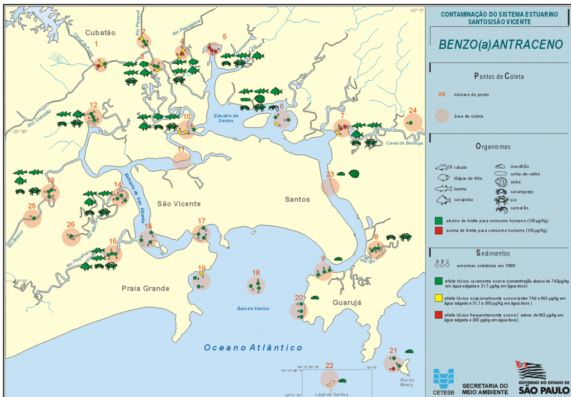
Figura 33- Mapa da contaminação por Benzo (a) Antraceno na Baixada Santista em 1999.
