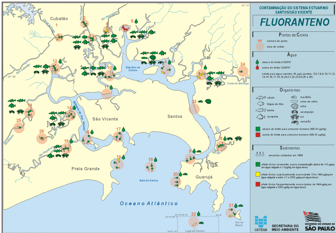
Figura 38- Mapa da contaminação por Fluoranteno na Baixada Santista em 1999.
