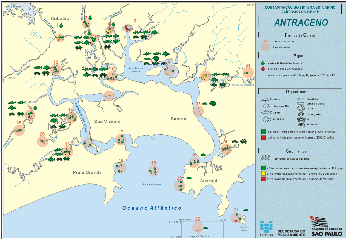
Figura 32- Mapa da contaminação por Antraceno na Baixada Santista em 1999.
