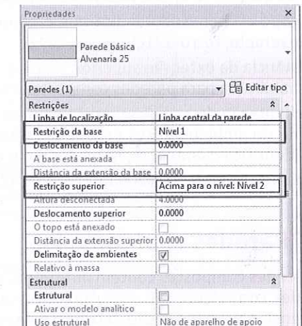
Figura 5.43 – Parede com altura até o Nível 2.
