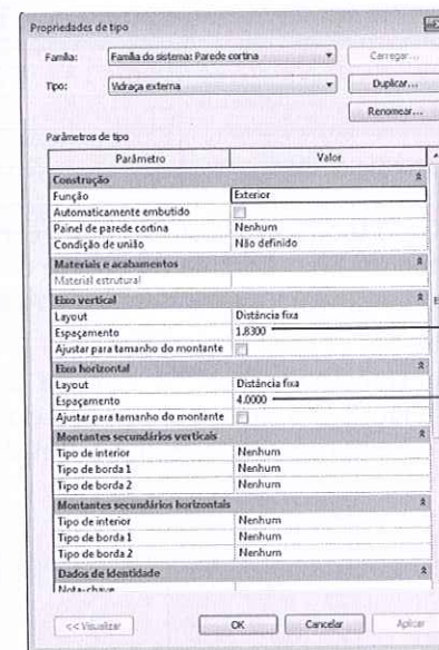
Figura 13.8 – Propriedades da parede Vidraça externa.
