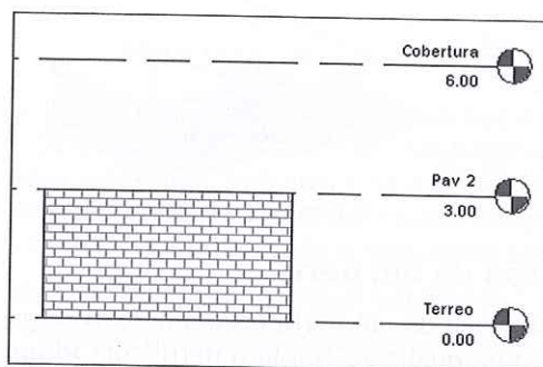
Figura 12.12 – Vista Leste.
