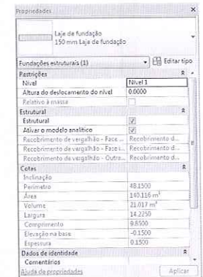
Figura 10.75 – Propriedades de instância da laje.
