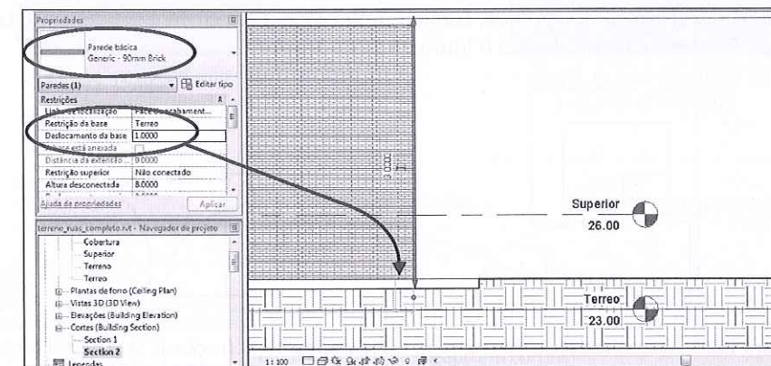
Figura 14.56 – Altura da base da parede igual à da base da plataforma.
