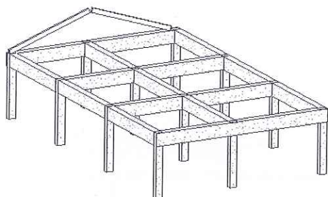
Figura 10.61 – Viga inclinada.
