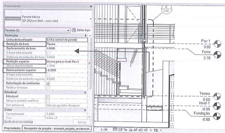
Figura 1.2 – Exemplo da parede associada ao pavimento.
