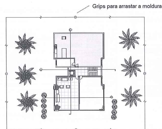
Figura 7.63 – Grips de corte da vista.
