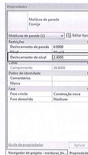
Figura 5.113 – Edição da altura da moldura.
