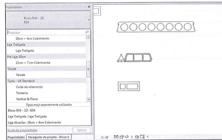
Figura 15.133 – Inserção de Componentes de detalhe.
