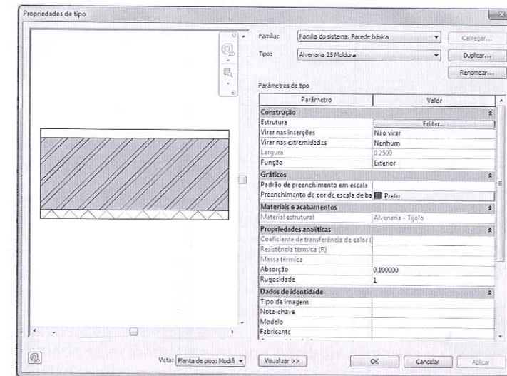
Figura 5.66 – Propriedades da estrutura da parede.
