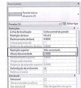
Figura 5.44 – Parede com altura fixa de 1 m.
