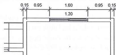
Figura 15.46 – Cota do peitoril da janela.
