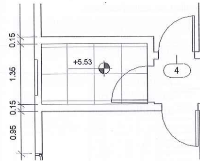
Figura 15.76 – Inserção de identificador em porta.
