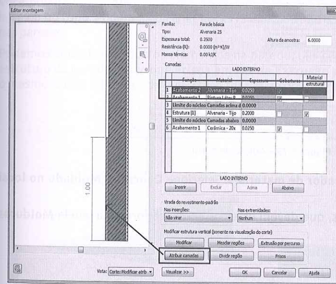
Figura 5.76 – Nova camada inserida.
