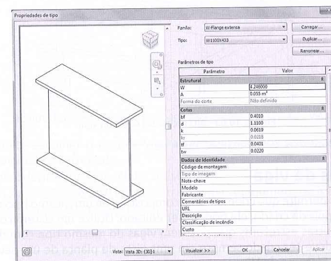
Figura 10.60 – Propriedades de viga metálica.
