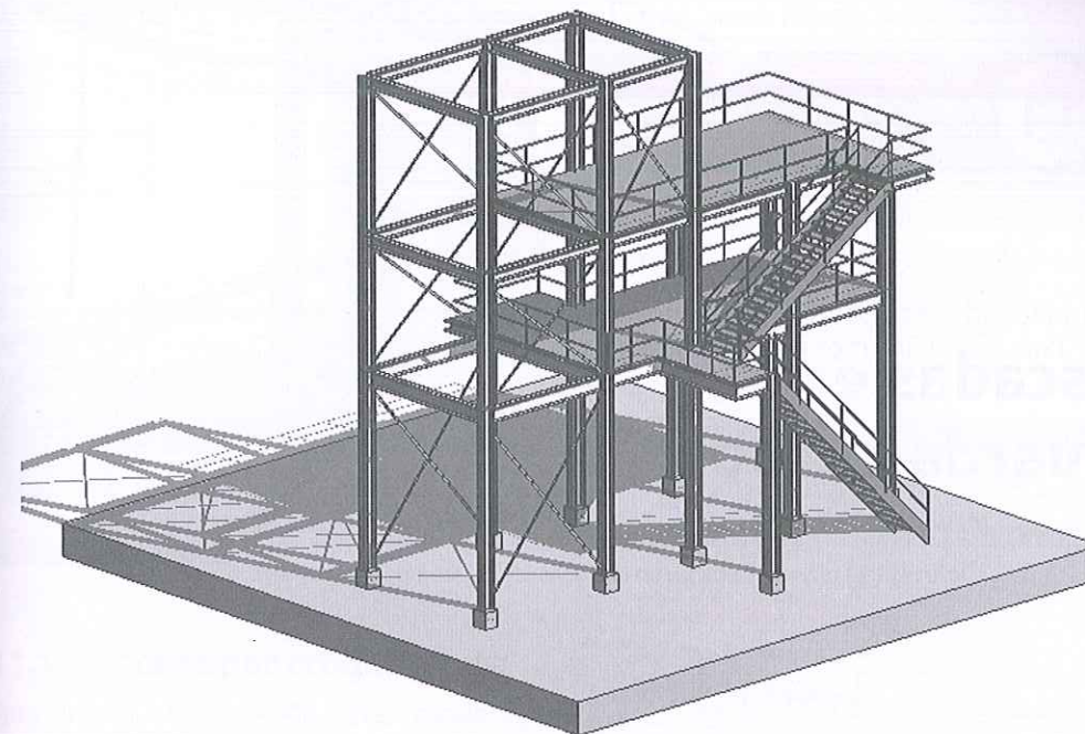
Figura 10.79 – Estrutura metálica.
