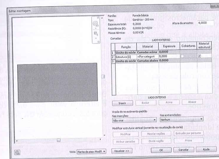
Figura 5.35 – Exemplo de estrutura de uma parede simples.
