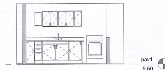
Figura 7.26 – Resultado da vista de elevação criada neste exemplo.
