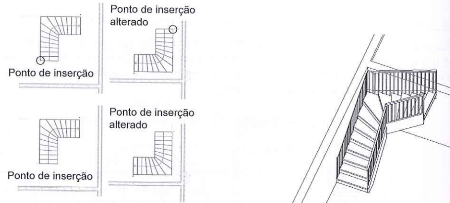
Figura 11.77 – Escada com degraus em leque.
