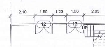
Figura 15.23 – Cotas alinhadas com aberturas.
