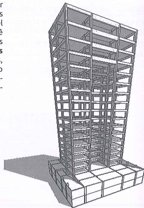
Figura 10.78 – Estrutura com pilares, vigas e lajes.
