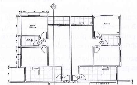
Figura 15.79 – Identificadores inseridos em todas as portas.
