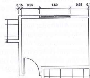
Figura 15.20 – Cotas alinhadas e na abertura da janela.
