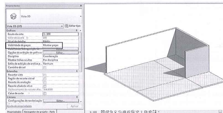
Figura 9.55 – Visualização das partes criadas.
