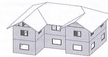
Figura 12.35 – Vistas do telhado após a eliminação de uma água.
