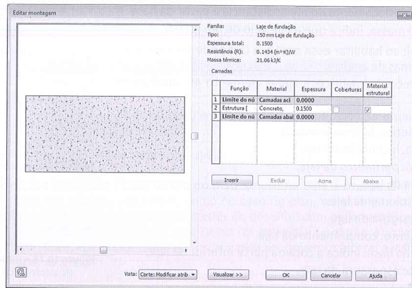
Figura 10.77 – Definição da estrutura da laje.
