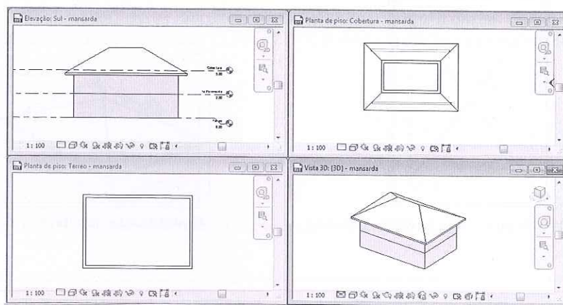
Figura 12.84 – Criação do telhado no pavimento da cobertura.
