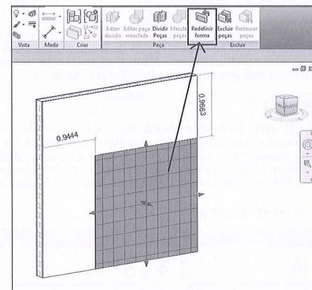
Figura 5.129 – Redefinir forma – desfazer a edição das partes.
