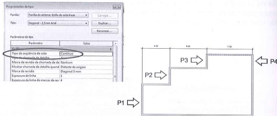
Figura 15.38 – Cota Contínuo.
