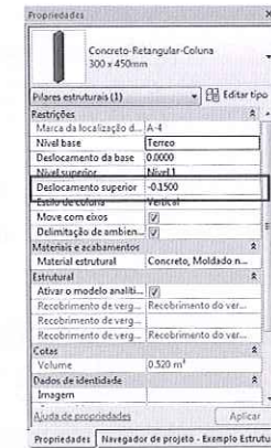
Figura 10.37 – Propriedades do pilar desassociado do piso.
