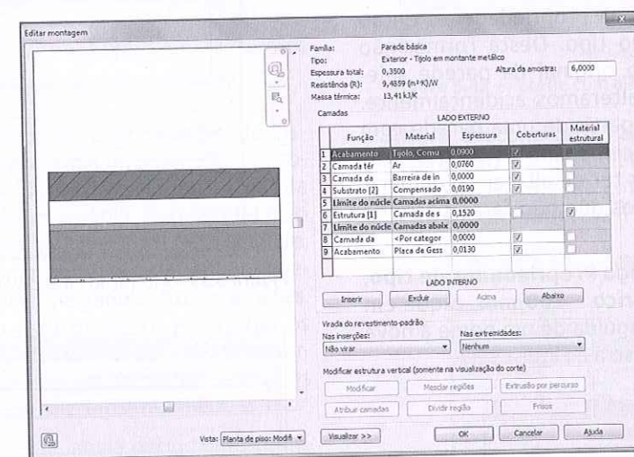
Figura 5.36 – Exemplo de estrutura de uma parede com várias camadas.
