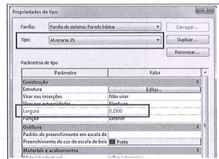
Figura 5.40 – Espessura alterada para 0.25.
