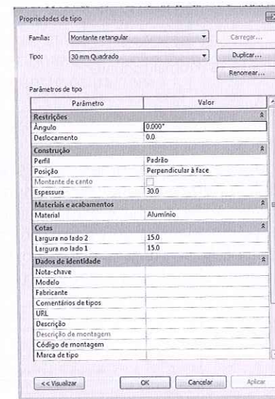
Figura 13.29 – Propriedades de tipo do montante.
