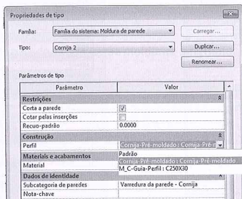
Figura 5.116 – Aplicando novo perfil.
