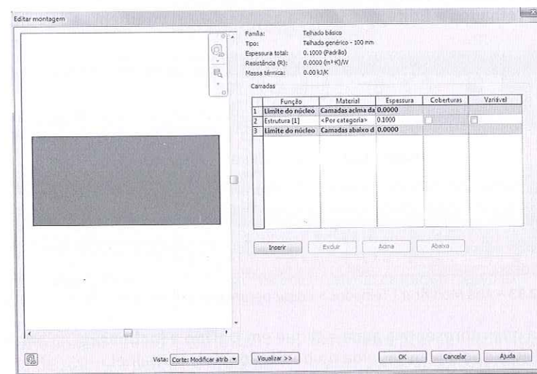
Figura 12.30 – Definição da estrutura do telhado.
