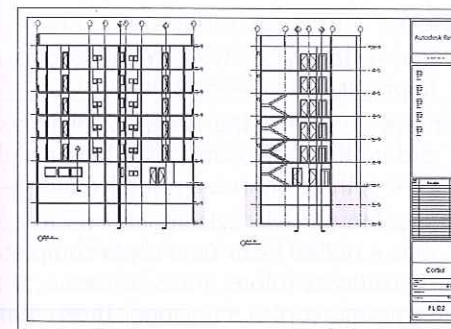
Figura 17.25 - Cortes.
