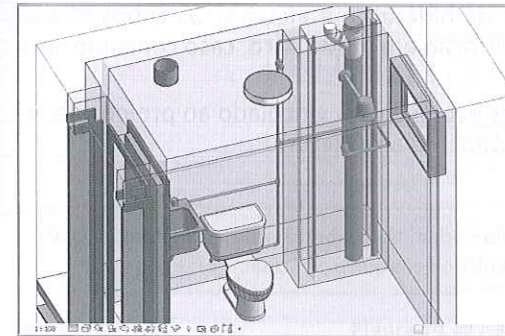
Figura 19.34 – Exemplo de projeto de instalações vinculado à arquitetura.
