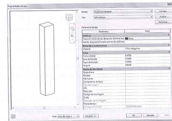
Figura 10.12 – Propriedades de tipo do pilar (Coluna: arquitetura).
