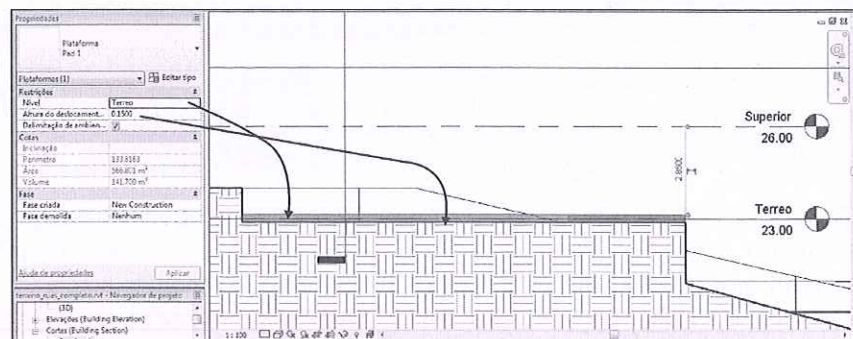
Figura 14.53 – Alteração da distância da plataforma ao pavimento térreo.
