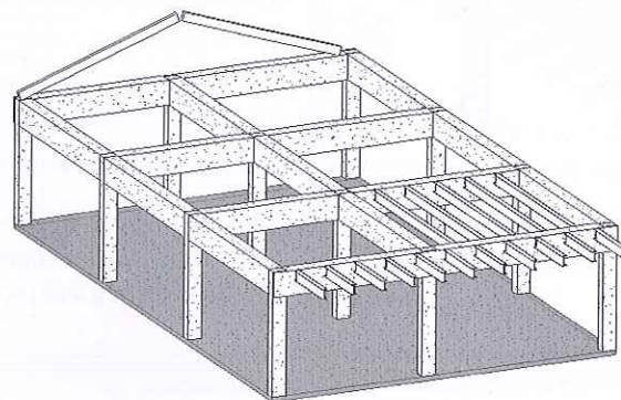
Figura 10.74 – Laje de fundação inserida.
