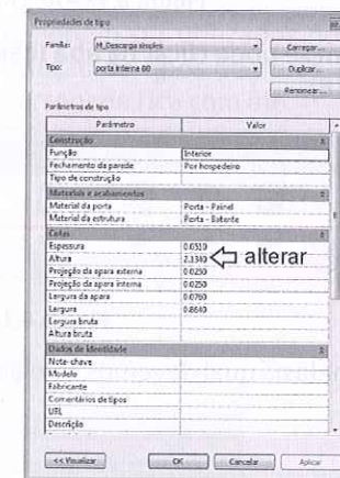
Figura 8.14 – Porta criada – porta interna 80.
