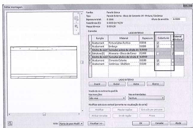
Figura 5.53 – Modificação do envolvimento pela edição da estrutura da parede.
