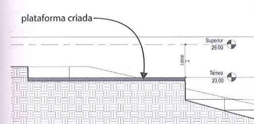
Figura 14.50 – Resultado da plataforma em corte.
