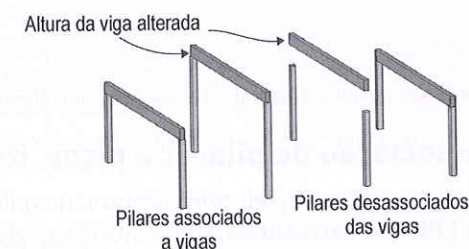
Figura 10.28 – Alteração da altura de vigas com pilares associados a elas e não associados.
