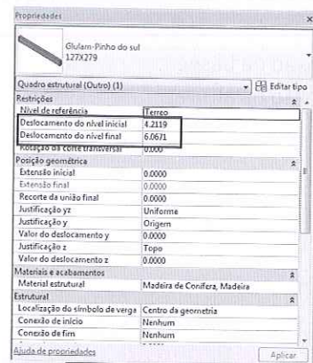
Figura 10.62 – Alturas das vigas.
