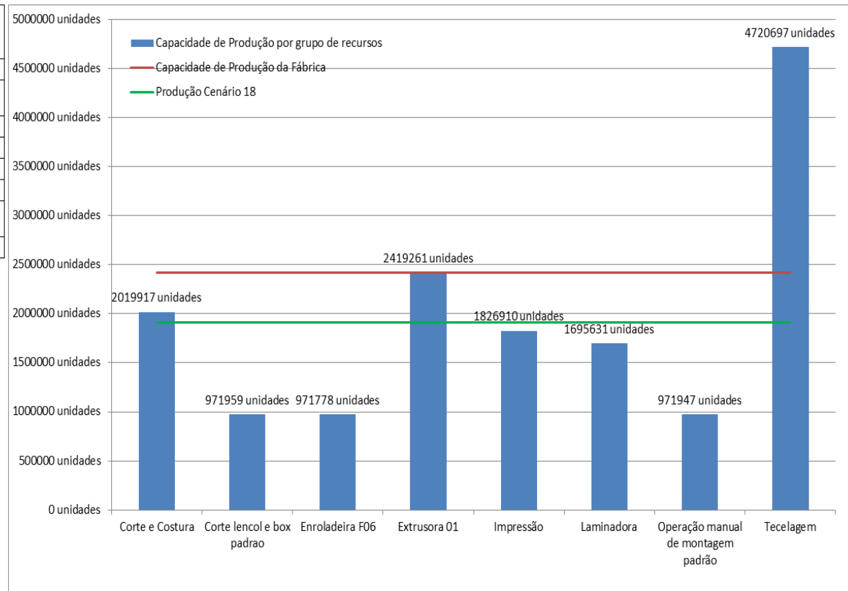
Figura 4.312 – Cenário 18 – Capacidade de Produção – Representação gráfica – réplicas 1 a 15. Fonte: Próprio autor.
