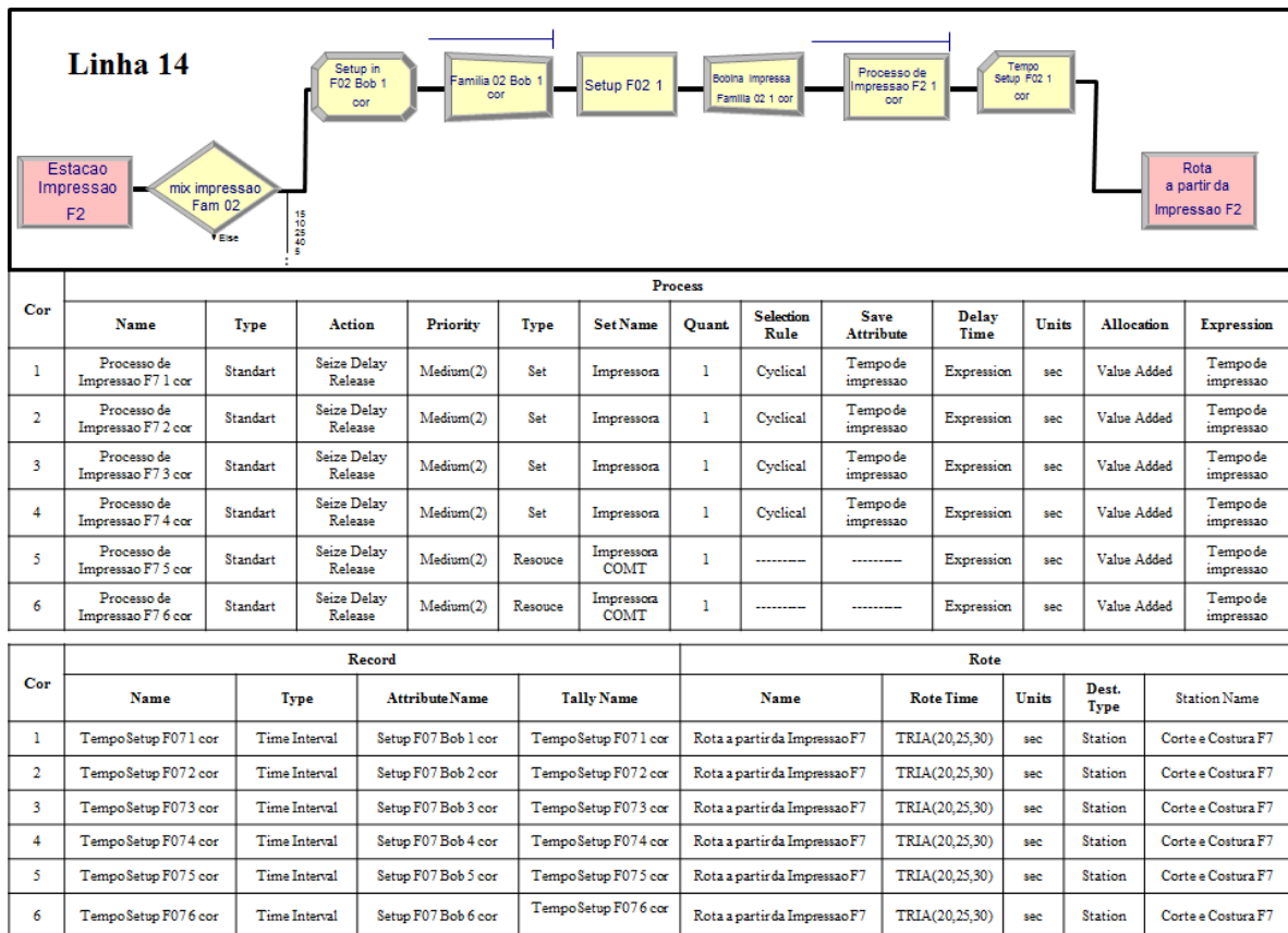
Figura 3.49 – Fluxo de produção do processo de impressão – setup – Família 7. Fonte: Próprio autor.
