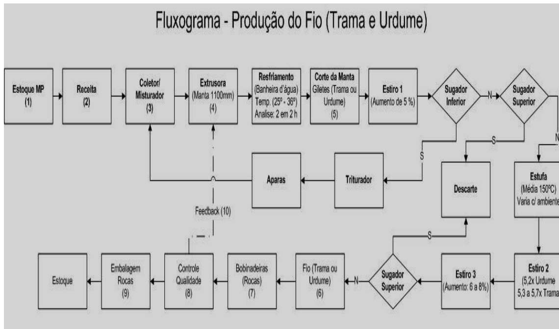
Figura 3.3 - Fluxograma da produção das fitas. Fonte: Emerson Marcos Minotti (2011).
