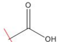
Ácido carboxílico
