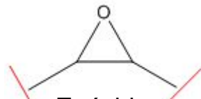
Epóxido
