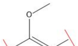
Enol-éter
