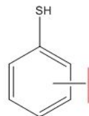
Tiofenol
