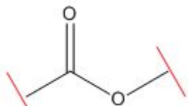
Éster
