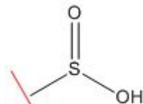
Ácido Sulfínico
