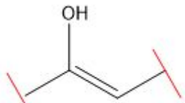
Enol
