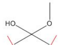
Hemiacetal
