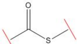
Tioéster
