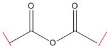
Anidrido
