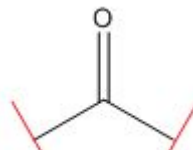
Cetona
