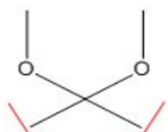
Acetal
