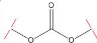
Carbonato
