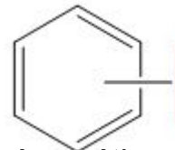
Aromático
