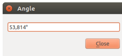
Figura11.22: Medir Ângulo
