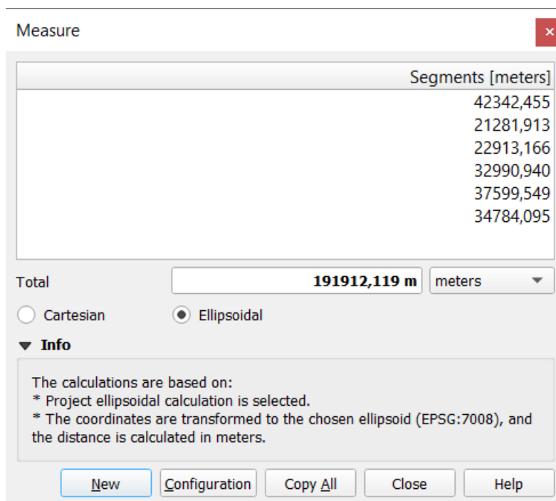
Figura 11.19: Medir Distância
