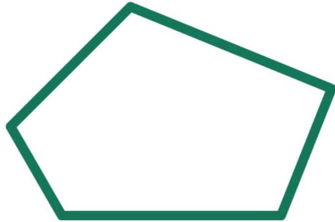
Polígono Convexo
