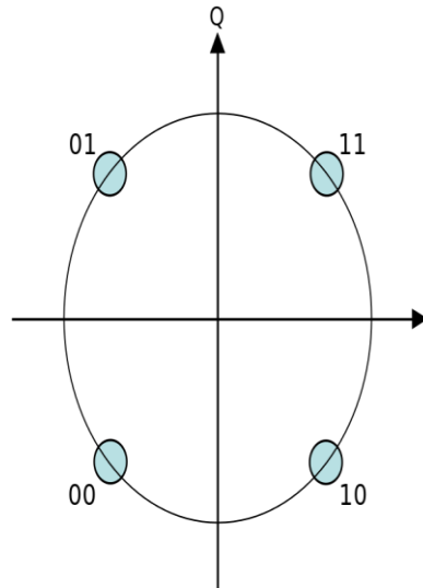
QPSK (4-PSK) quadrature
