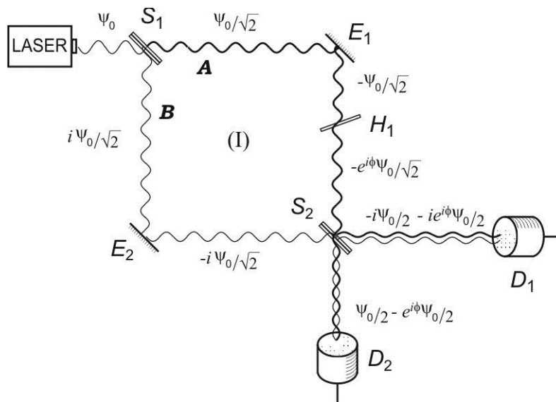
Figura V.1. Interferômetro de Mach-Zehnder, com as amplitudes clássicas em cada trecho.
