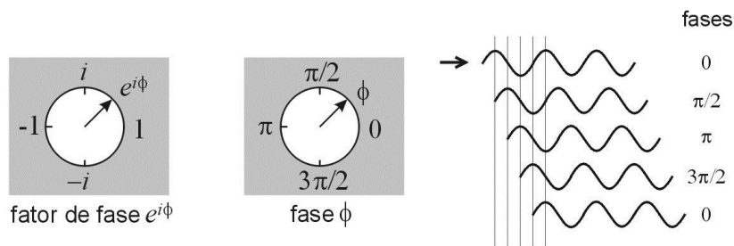
Figura V.2: As fases relativas entre ondas contínuas são expressas por ângulos em radianos, como \pi/2 , \pi , 3\pi/2 e 2\pi , que denotam respectivamente avanços de 1/4 de ciclo, 1/2 ciclo, 3/4 de ciclo e um ciclo inteiro. Este último é equivalente à fase da própria onda original, no caso de ondas contínuas. Cada fase \phi , então, pode ser representada como uma direção de um círculo. Mas os números complexos também permitem uma representação elegante dessas fases, por meio do fator de fase e^{i\phi} , multiplicado ao valor da amplitude.
