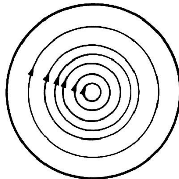
TE_{01}
