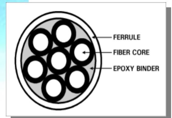
Seção Transversal de um cabo óptico
