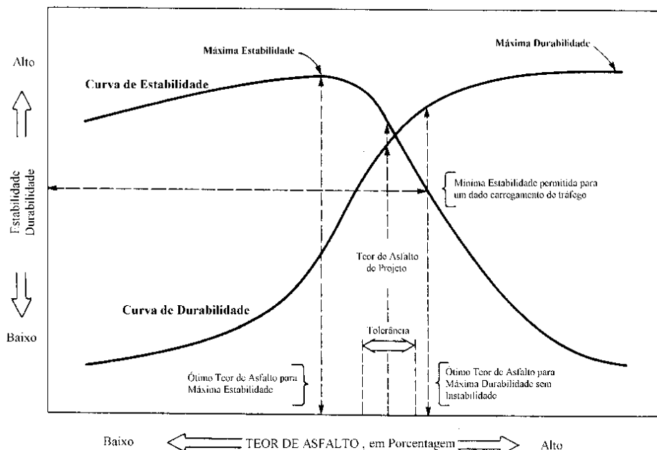
Figura 1: Variação de propriedades de misturas asfálticas com o teor de ligante
