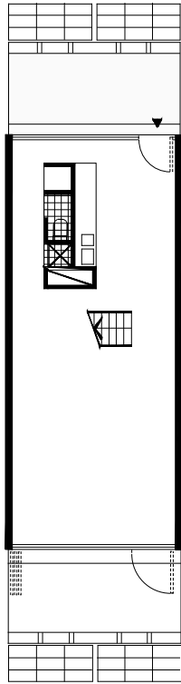
Planta baixa do apto triplex - Nível inferior ou de acesso
