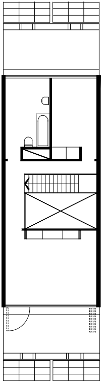
Planta baixa do apto triplex - Nível superior
