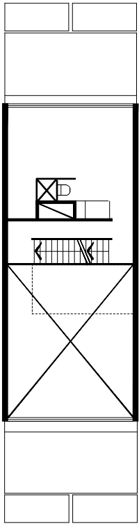
Planta baixa do apto triplex - Nível intermediário
