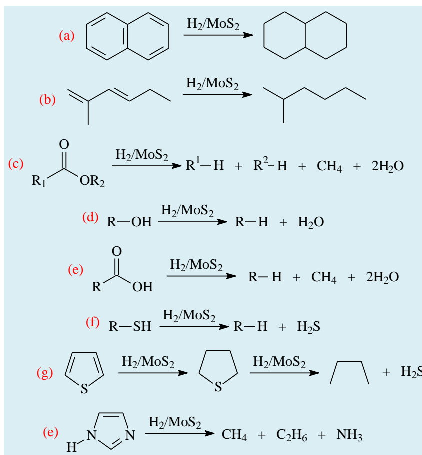
Figura 10. Reações de hidrogenação realizadas na indústria do petróleo para produzir combustíveis: (a) desaromatização; (b) eliminação de olefinas; eliminação de oxigênio de ésteres (c), alcoóis (d) e ácidos carboxílicos (e); dessulfurização de mercaptanas (f) e tiofeno e tioéter (g); e (e) desnitrogenação de aminas
