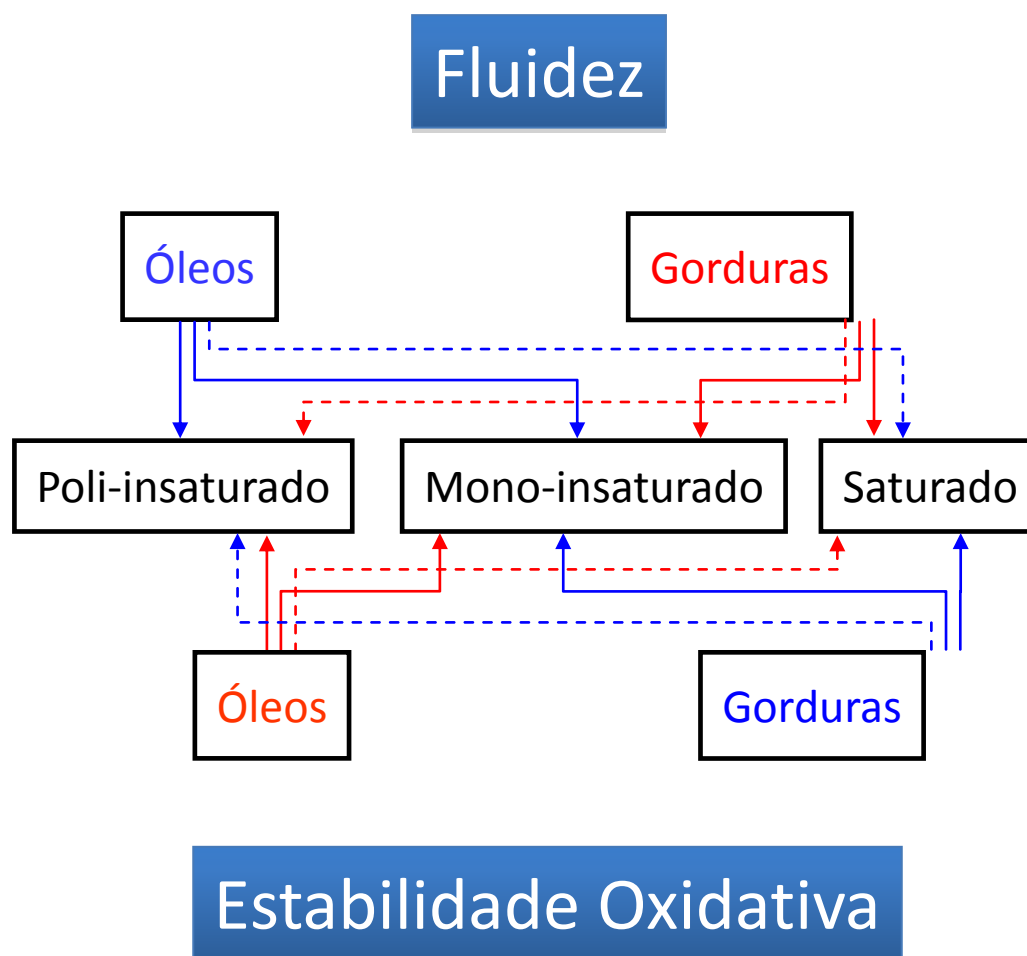
Figura 3. Influencia das ligações duplas nas propriedades físicas e químicas de óleos e gorduras: enquanto cadeias saturadas (gorduras) favorecem a estabilidade oxidativa, comprometem a fluidez do material graxo, sendo exatamente o contrário para as cadeias poli-insaturadas (óleos)
