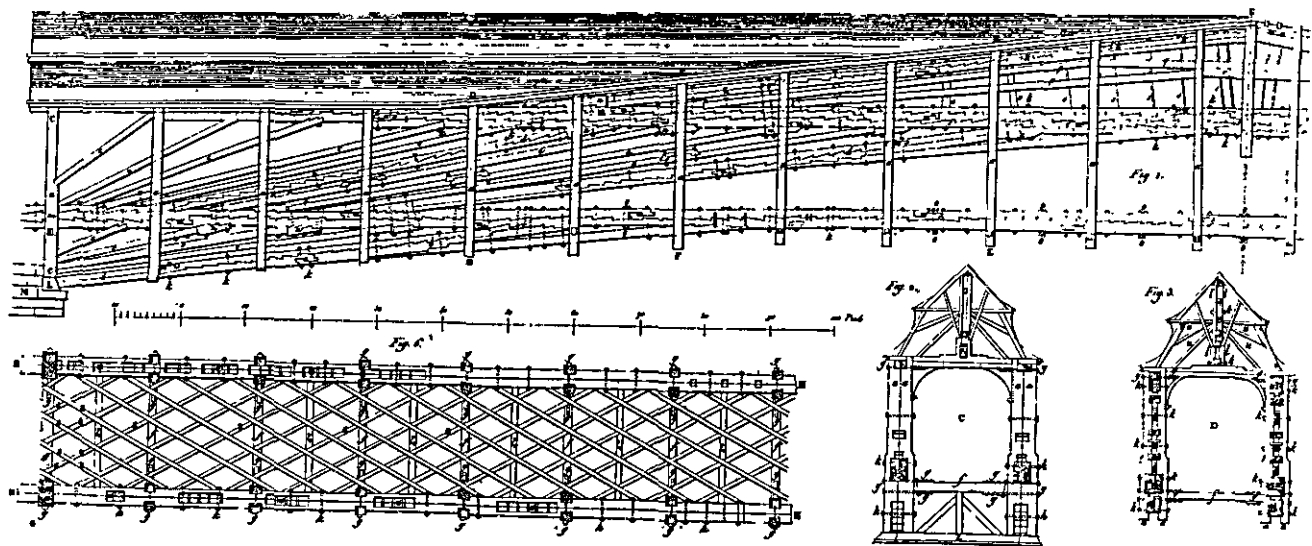
15. A ponte sobre o rio Limmat em Wettingen (J. U. Grubemann, 1777; em Trattato , de G. Rondelet, prancha 103). 16. Representação do corte das pedras (do Trattato de G. Rondelet, prancha 40).
