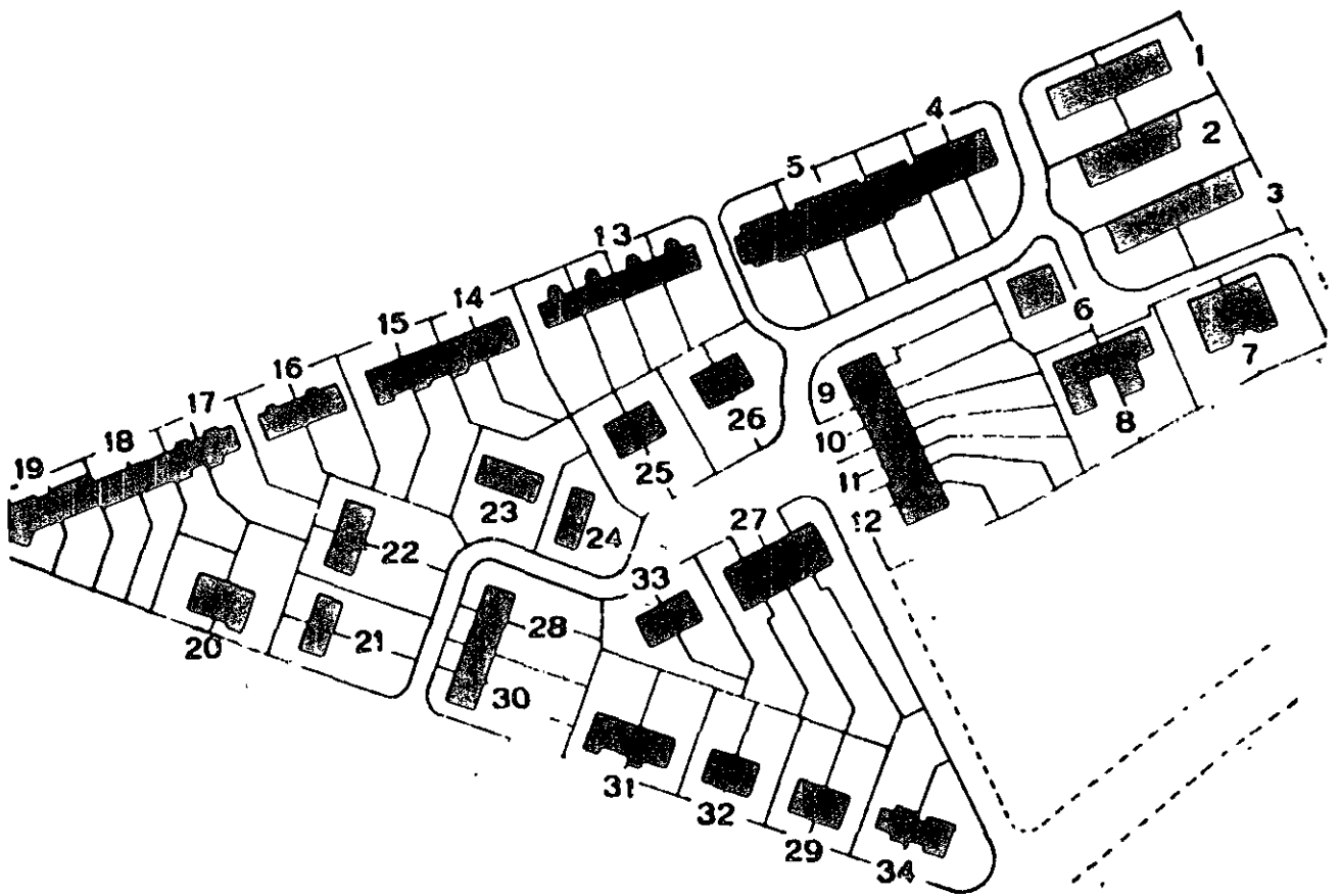
669. Viena, Werkbundsiedlung de 1932, planimetria geral.
