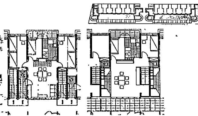
511-515. Hock van Holland, as duas casas geminadas de J. J. P. Oud, 1924; o tipo da construção, a planimetria e três vistas recentes.
