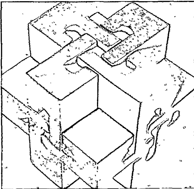
805-808. Detalhes do packaged house system estudado por Gropius e Wachsmann em 1942, para a General Panel Corp. (de K. W., The Turning Point of Building ).
