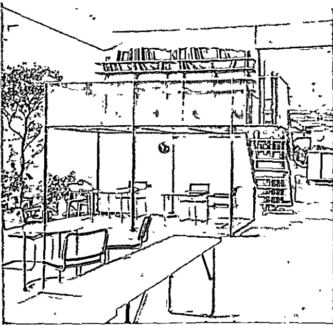
554, 555, 556. Berlim, Bauausstellung 1931: em cima, decoração de L. Reich; embaixo a planta e uma vista de casa-modelo de Mies van der Rohe (de P. Johnson, op. cit.).
