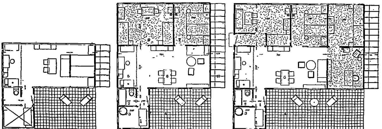
606, 607. W. Gropius, a casa alta estudada para o bairro de Spandau de 1929 e a casa pré-fabricada ampliável estudada para a Hirsch Kupfer und Messingwerke A. G. em 1931 (de S. Giedion, op. cit.).
