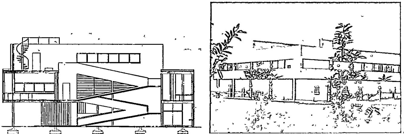
567, 568, 569. Poissy e Villa Savoye (seção e vista original da Oeuvre complète ).
