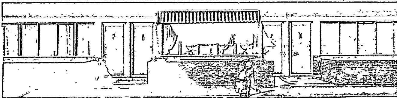
511-515. Hock van Holland, as duas casas geminadas de J. J. P. Oud, 1924; o tipo da construção, a planimetria e três vistas recentes.
