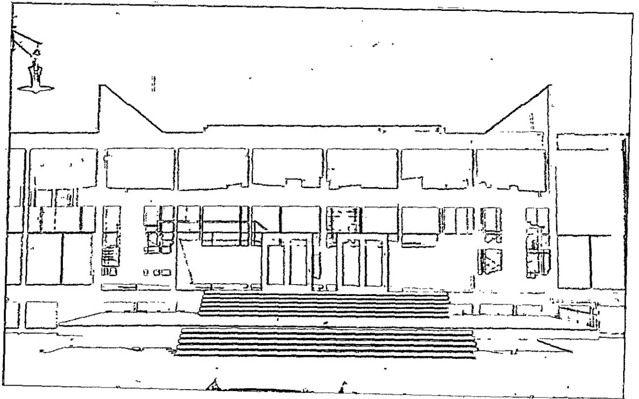
816, 817, 818. Chicago, o Crown Hall (Mies van der Rohe, 1955; planta de P. Johnson, M. v. d. R. ).
