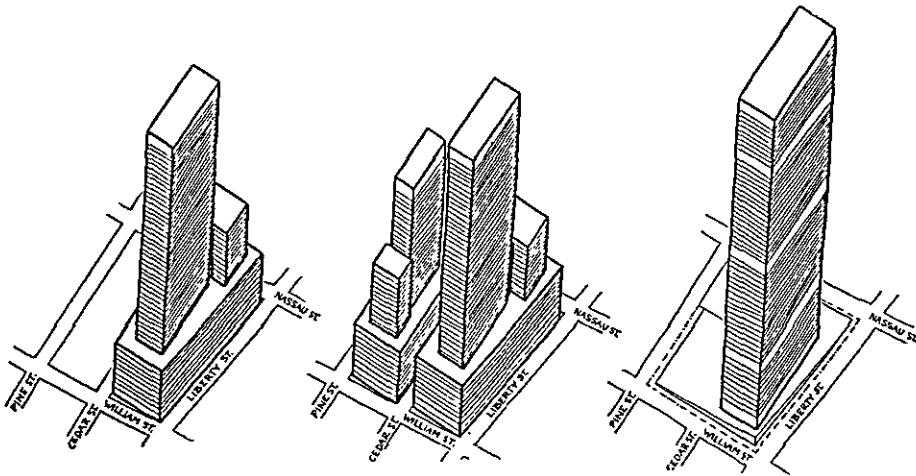
1014, 1015. O Chase Manhattan Building de Nova York, com as três soluções volumétricas apresentadas por Skidmore, Owings & Merrill aos clientes. 1016. Chicago, o campus do IIT, com o Crow Hall e os novos edifícios de Skidmore, Owings e Merrill, sobre o fundo do centro da cidade.
