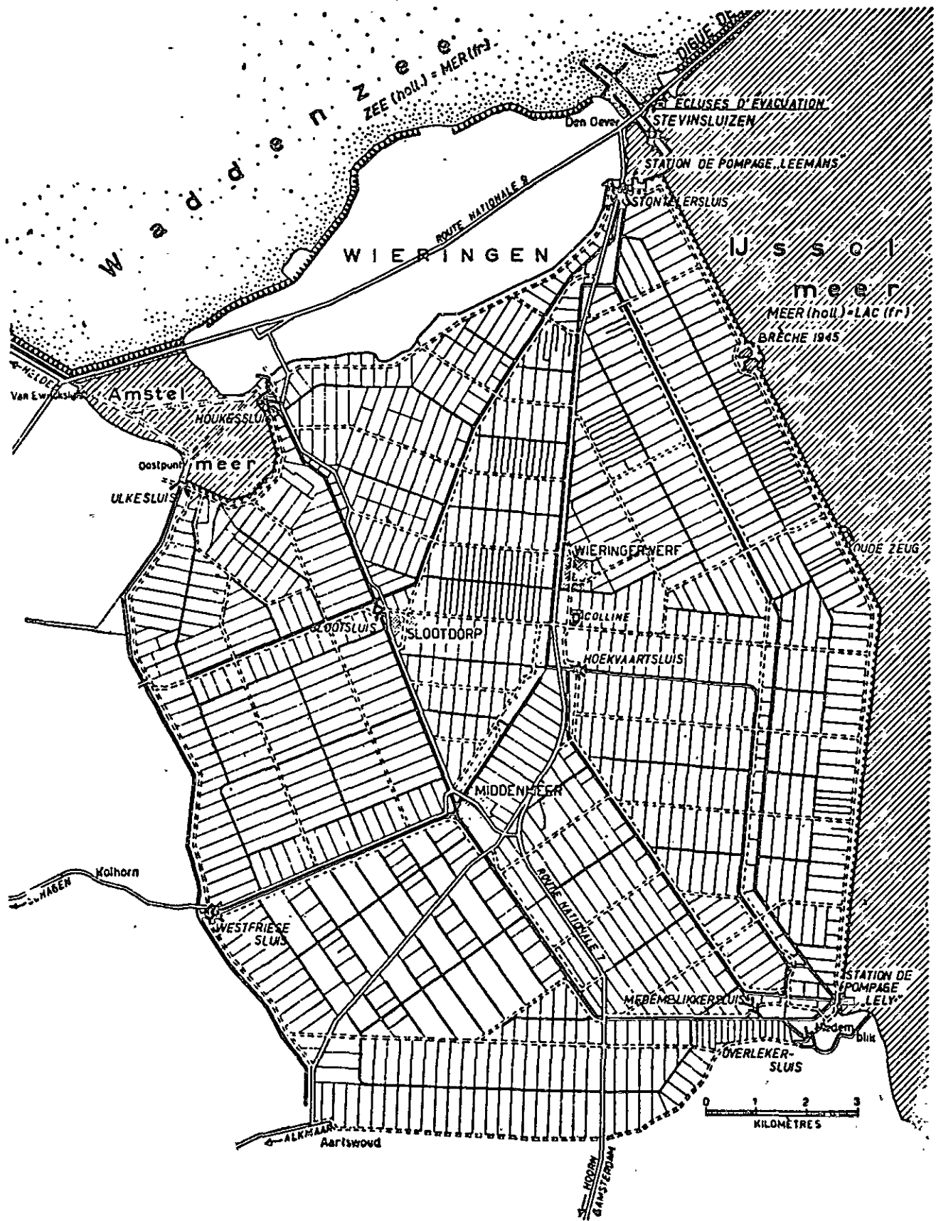
942. Plano de adaptação do terreno do polder de Wieringermeer (em traços pretos grossos, os canais; de Urbanística).
