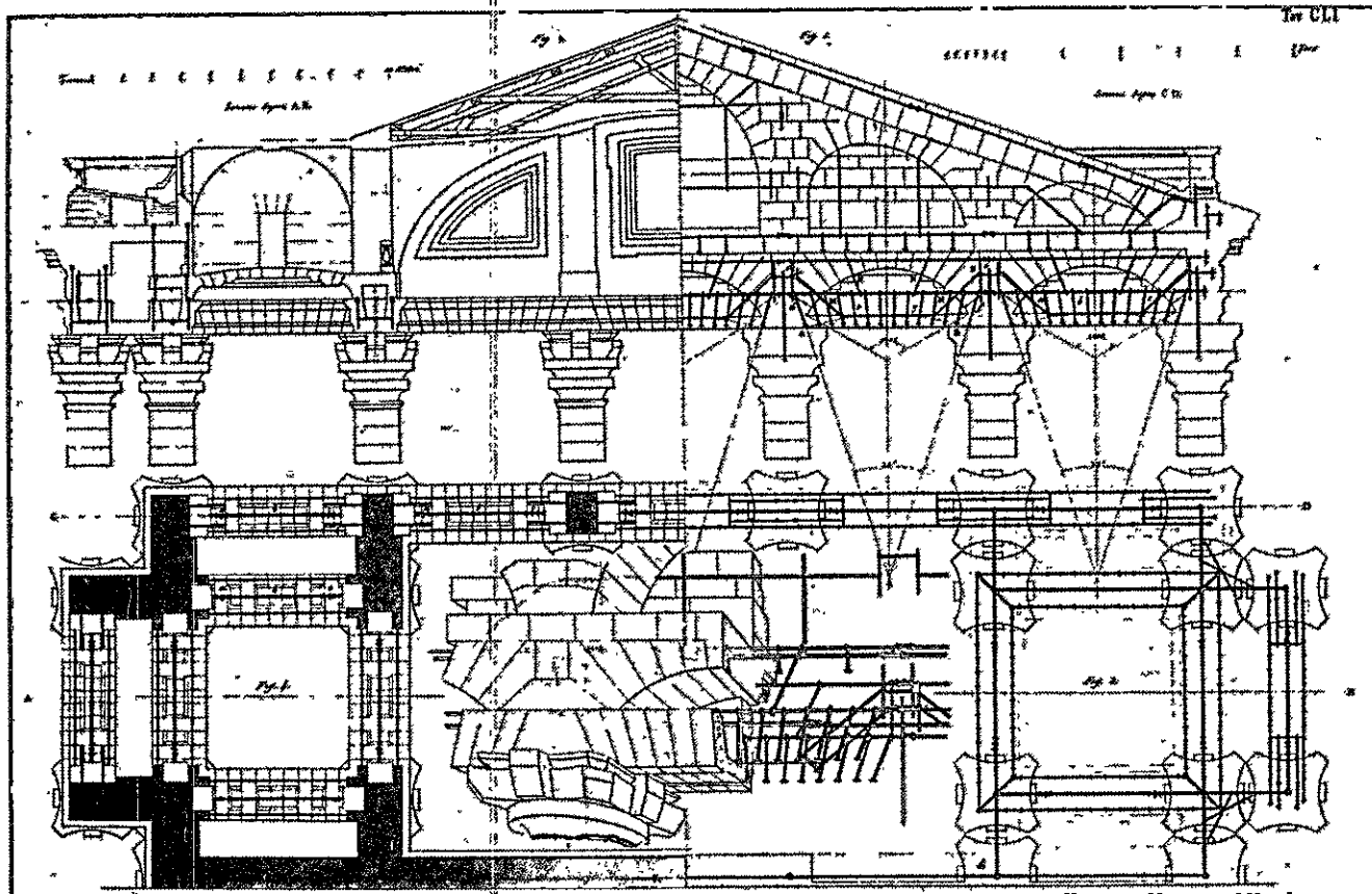
19, 20, 21. Paris, a igreja de Sainte-Geneviève (J. G. Soufflot, 1755): a armação em ferro da pronave (do Trattato de G. Rondelet, planca 151), a planta e a fachada.
