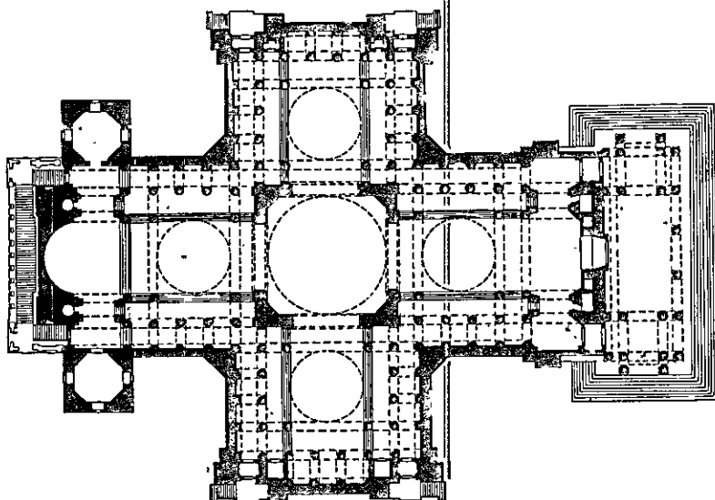
19, 20, 21. Paris, a igreja de Sainte-Geneviève (J. G. Soufflot, 1755): a armação em ferro da pronave (do Trattato de G. Rondelet, planca 151), a planta e a fachada.
