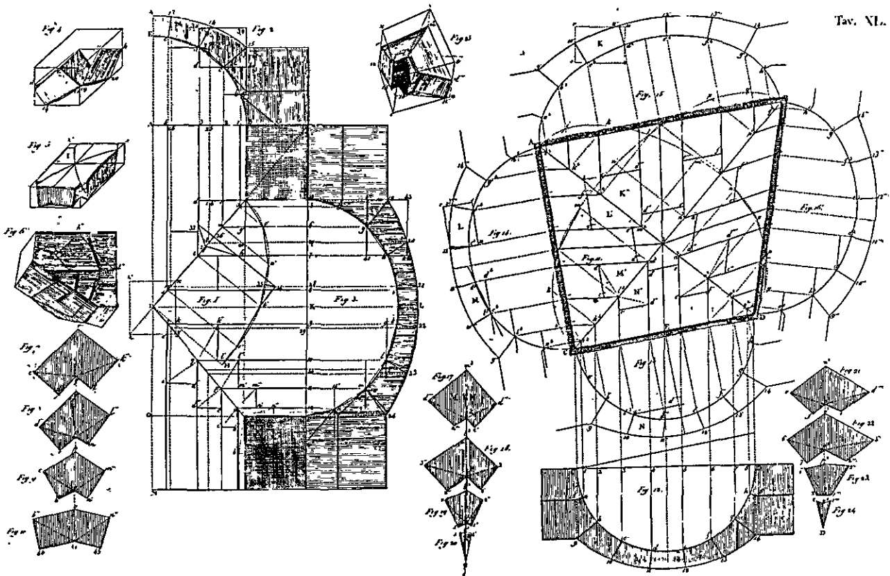
15. A ponte sobre o rio Limmat em Wettingen (J. U. Grubemann, 1777; em Trattato , de G. Rondelet, prancha 103). 16. Representação do corte das pedras (do Trattato de G. Rondelet, prancha 40).
