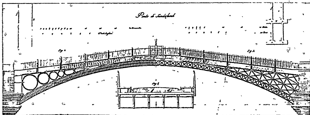
22, 23. A ponte sobre o Severn em Coalbrookdale (T. F. Pritchard 1777) e a ponte sobre o Wear em Sunderland (R. Burdon, 1796; do Trattato de G. Rondelet, pranchas 157 e 158).
