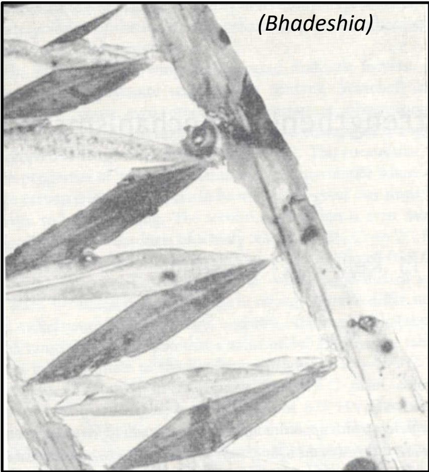
MARTENSITA MACLADA
