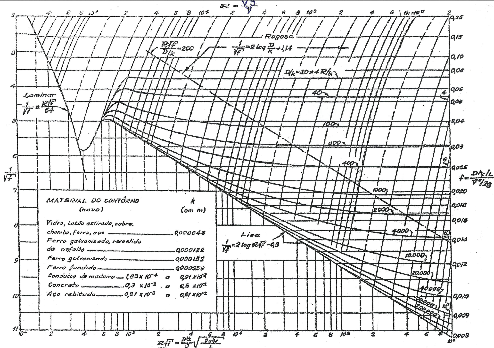
DIAGRAMA de MOODY-ROUSE
