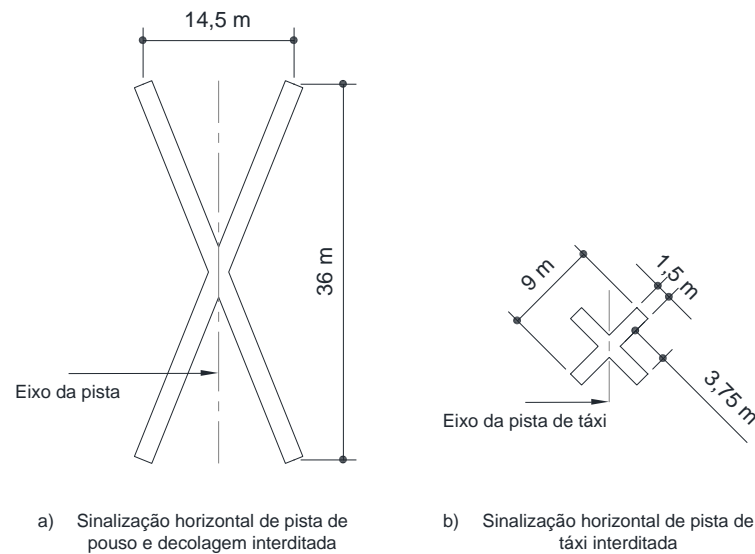
Figura E-1. Sinalizações horizontais de pistas de pouso e decolagem e de pista de táxi interdidadas (Alterado pela Resolução nº 465, de 13.03.2018)
