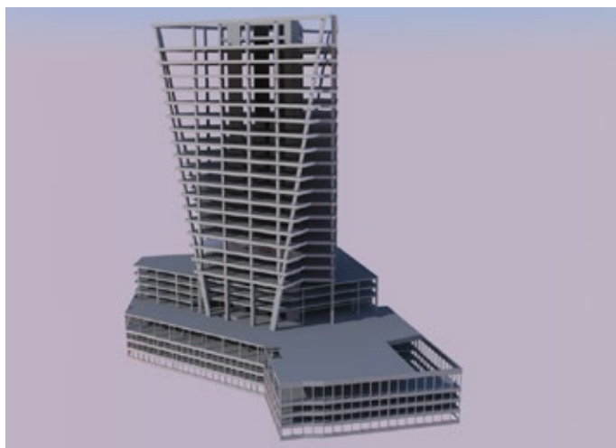
Figura 92: Estrutura modelada, calculada, detalhada e documentada com o software TQS (Ávila Engenharia de Estruturas – Marília – SP)
