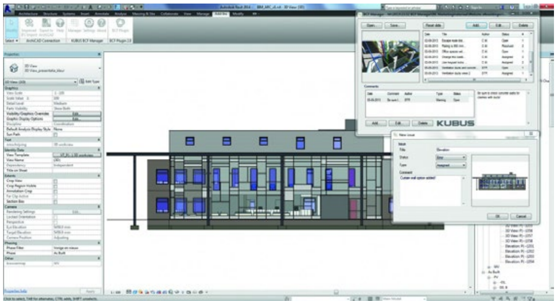
Figura 62: Ilustração demonstrando a identificação de uma interferência no software Revit, com a gravação de um arquivo formato BCF xml, instalado pelo plug-in Kubus, registrando o ângulo de visão no momento em que o problema foi identificado e a inclusão de anotações por parte do usuário que a fez
