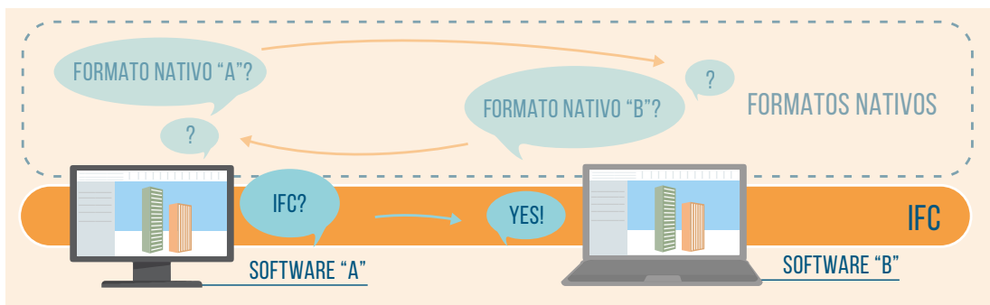
Figura 56: Dois softwares diferentes talvez não consigam se comunicar utilizando seus formatos nativos, mas talvez possam se comunicar utilizando um formato ‘neutro’ como o IFC
