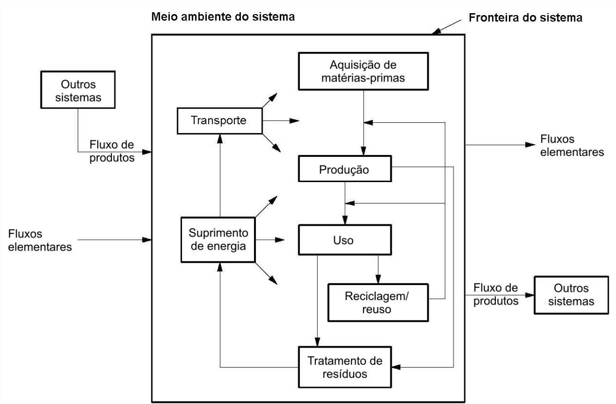
Figura 2 — Exemplo de um sistema de produto para ACV
