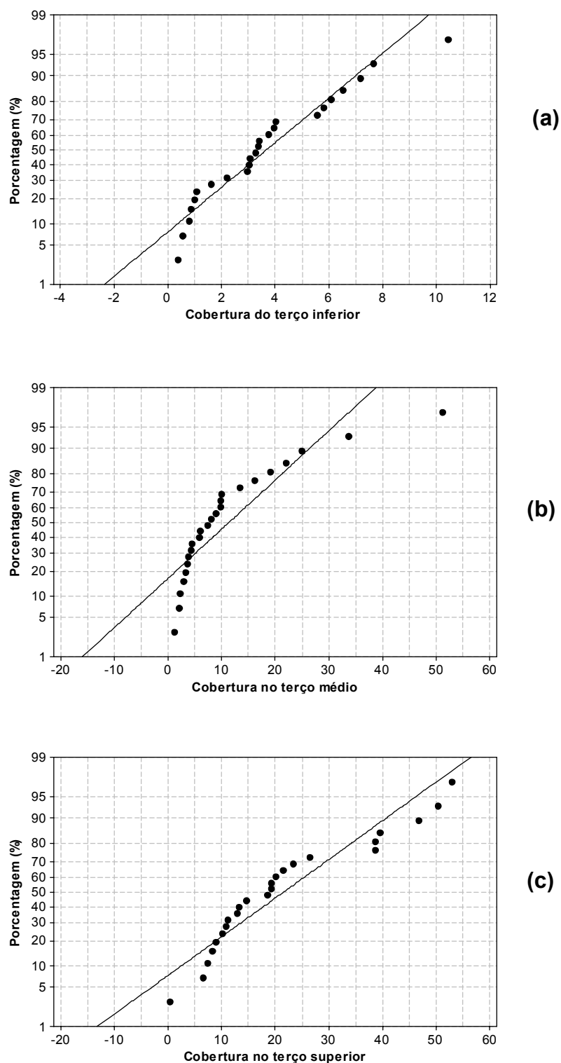
FIGURA 1 – Teste de normalidade para porcentagem de cobertura por pontas de jato plano duplo e jato cônico nos terços inferior (a), médio (b) e superior (c) da planta de soja.
