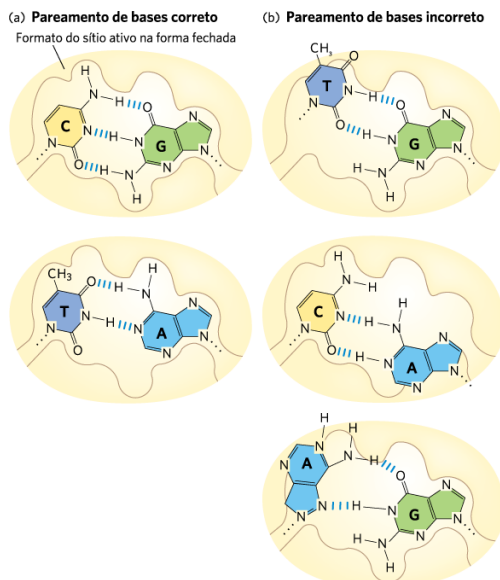
FIGURA 11-10 Pareamento de bases na cavidade do sítio ativo de Pol I. (a) O formato do sítio ativo na conformação fechada. Pares de bases corretos G=C e A=T ajustam-se dentro do sítio ativo. (b) Pareamentos de bases incorretos não se encaixam no sítio.
