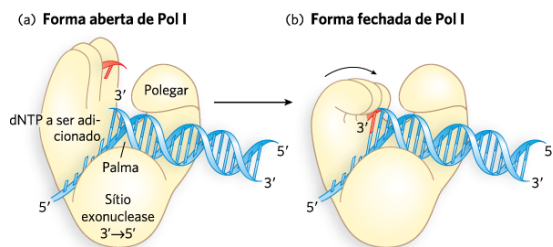
FIGURA 11-9 Formas aberta e fechada de Pol I. (a) Na forma aberta, um dNTP liga-se ao domínio dos dedos. (b) Na forma fechada, o domínio dos dedos sofre uma rotação de 40° que move o dNTP para dentro, na posição de pareamento de base com o molde, e constitui uma cavidade no sítio ativo que acomoda o formato de um pareamento de base Watson-Crick correto.
