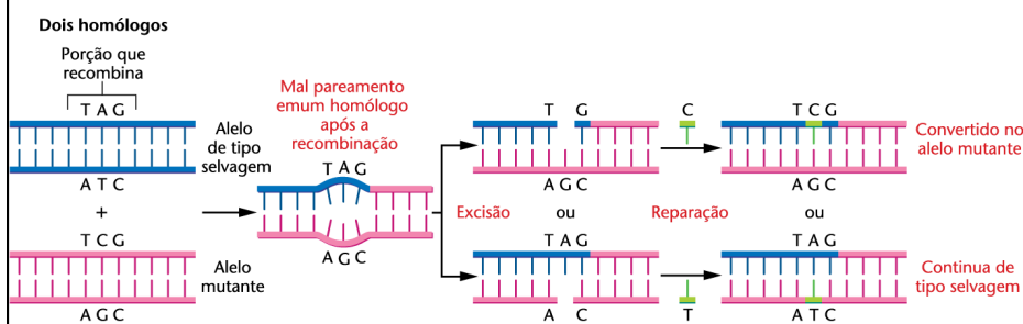
FIGURA 11-19 Proposta de um mecanismo responsável pelo fenômeno da conversão gênica durante a recombinação na meiose. Ocorre o mal pareamento de um par de bases em um homólogo recombinante (devido à presença de um alelo mutante) durante a formação do heterodúplex. Durante a reparação por excisão, uma das duas bases mal pareadas é removida, e o complemento é sintetizado. Em um caso, o par de bases mutante é preservado; quando é subsequentemente incluído em um esporo recombinante, o genótipo mutante será mantido. No outro caso, o par de bases mutante é convertido na sequência de tipo selvagem. Quando incluído em um esporo recombinante, o genótipo de tipo selvagem será expresso, causando uma proporção de troca não recíproca.
