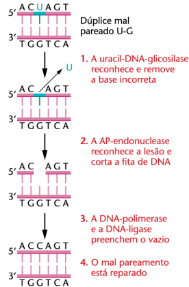
FIGURA 16-13 Reparação por excisão de base (BER) completada pela uracil-DNA-glicosilase, pela AP-endonuclease, pela DNA-polimerase e pela DNA-ligase. A uracila é reconhecida como uma base não complementar, é removida e substituída pela base comple-
