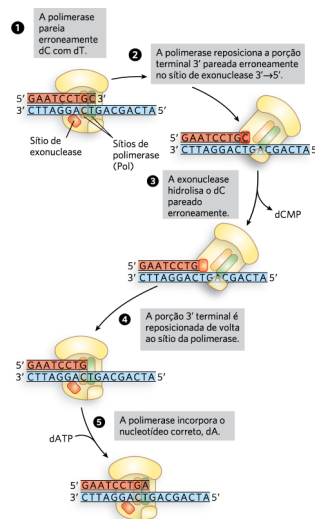
FIGURA 11-6 A atividade de exonuclease 3'-5' de correção de erro das DNA-polimerases. O sítio ativo da exonuclease 3'-5' é distinto do sítio de polimerização e revisa o produto da DNA-polimerase.
