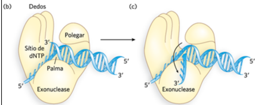
(c) Uma porção terminal 3' pareada erroneamente abre o espaço de cerca de 4 nucleotídeos para inserir-se dentro do sítio de exonuclease 3'→5'. [Fonte: (a) PDB ID 4KTQ.]
