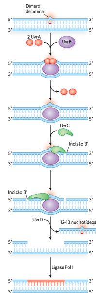
FIGURA 12-24 Reparo por excisão de nucleotídeos em E. coli . A via NER utiliza diversas proteínas, inclusive UvrA (vermelho), UvrB (roxo) e UvrC (verde), que reconhecem a lesão e produzem incisões em cada um dos lados, permitindo que a UvrD (helicase II) desloque uma parte do DNA com lesão. A lacuna na fita simples é preenchida pela Pol I, e o DNA é selado pela ligase. Um caminho de reparo acoplado à transcrição (TCR) pode ainda ser seguido, quando a RNA-polimerase trava em uma lesão na fita codificante. Depois que a RNA-polimerase é deslocada, a reação procede como demonstrado aqui, utilizando de UvrA a UvrD, Pol I e ligase.
