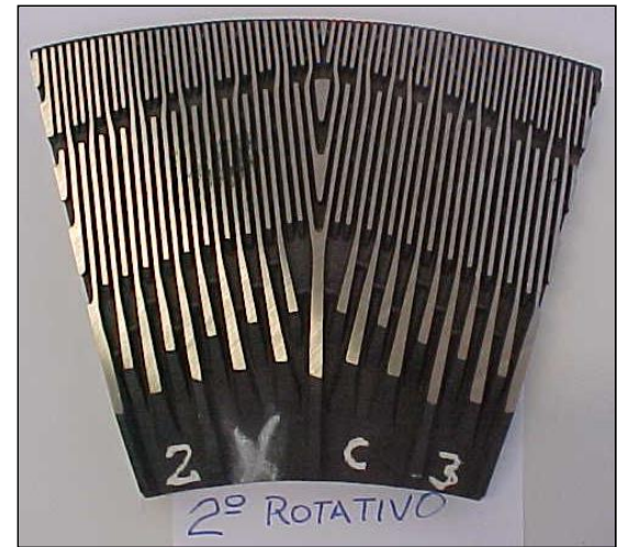
Figura 3. Ilustração de um refinador de discos (a) e fotografia de uma fração de um disco refinador (b) com as ranhuras responsáveis pela ação abrasiva sobre os cavacos de madeira.
