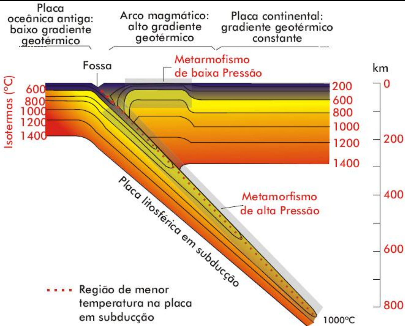
Fig. 18.20 Padrão das isotermas em uma zona de subducção.
