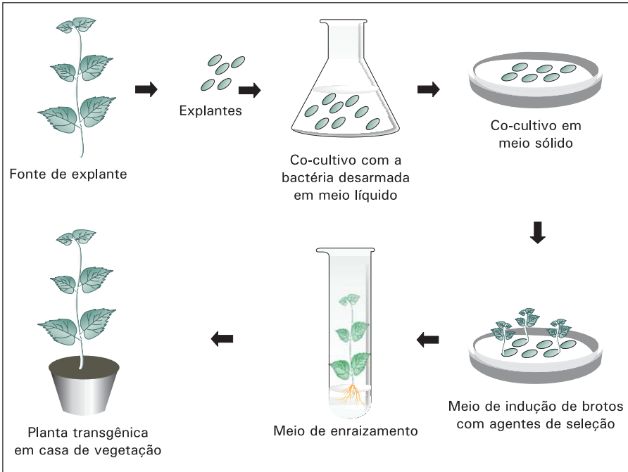
Figura 4. Transformação por Agrobacterium .
