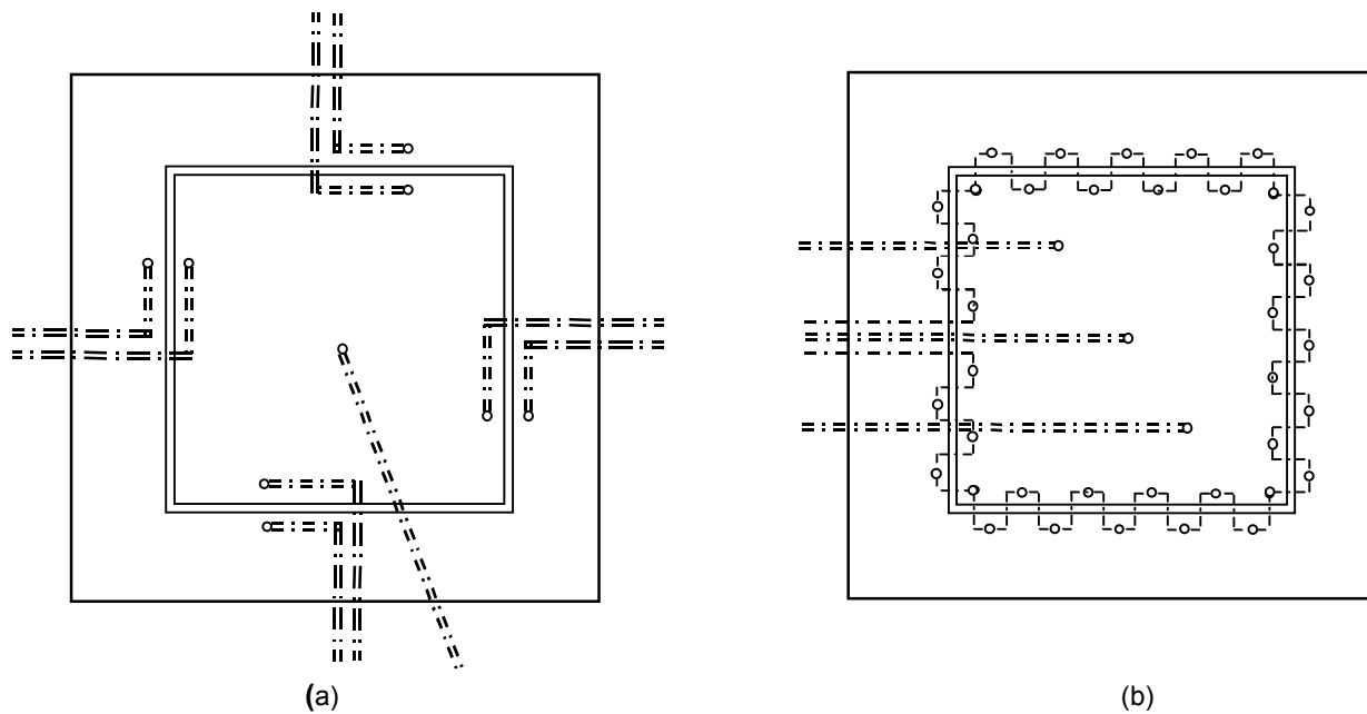
Figura 3 — Disposição dos termopares na placa quente
