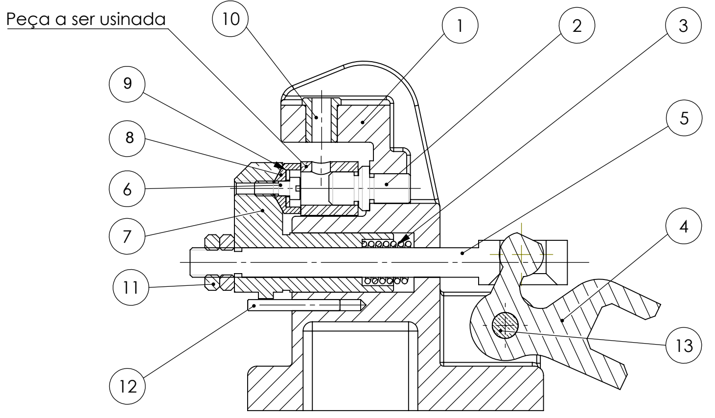
A-A (1 : 1)
