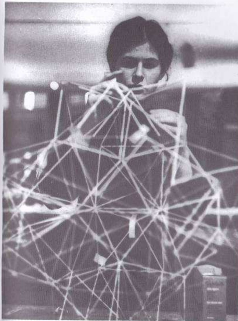
Uma aluna do Carpenter Center constrói uma estrutura tridimensional à base de triângulos equiláteros, utilizando um material muito frágil para melhor controlar a robustez do conjunto.
