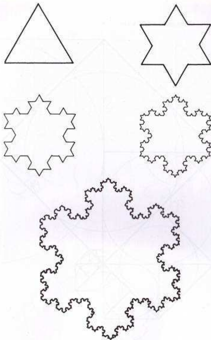
Dividindo-se em três partes cada lado de um triângulo equilátero e construindo um triângulo externo em cada lado, obtém-se a segunda figura. Continuando a operação em cada novo lado chega-se à chamada curva de floco de neve. É possível fazer a mesma operação, desenhando os triângulos no interior dos lados: a figura muda.
