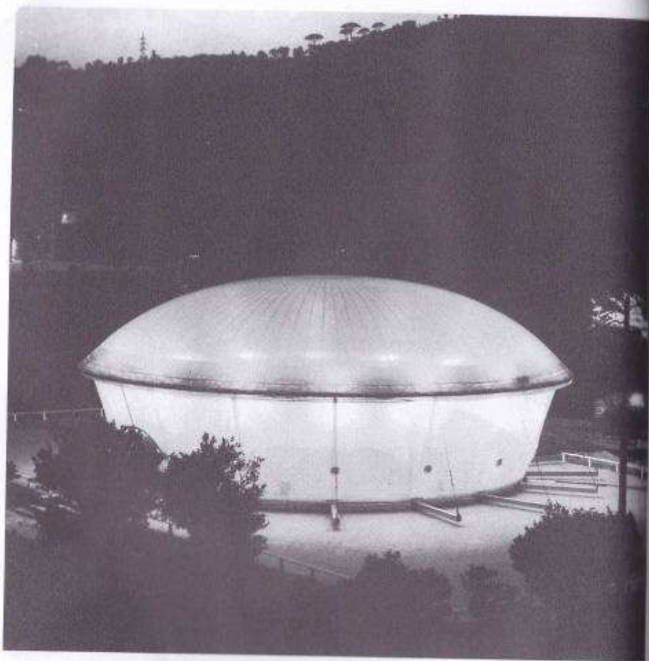
Pavilhão móvel com cúpula pressostática para a Radiotevisão Italiana, 1967. Design A. e P. G. Castiglioni.
