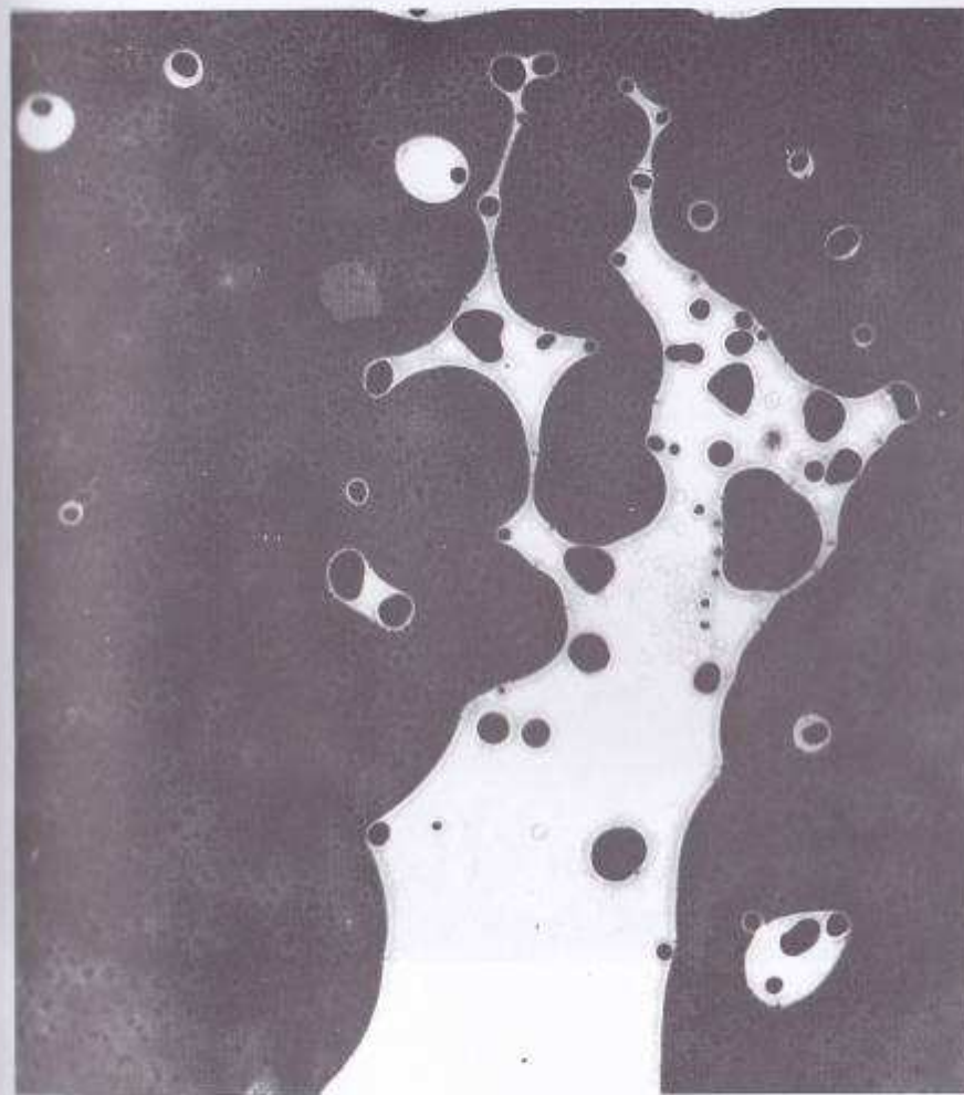
Formas naturais de combinação entre dois líquidos com densidades diferentes (água e óleo), no momento da passagem do estado de emulsão ao estado de isolamento. Imagens obtidas com termocopiadora, por Tonino Petrocelli.
