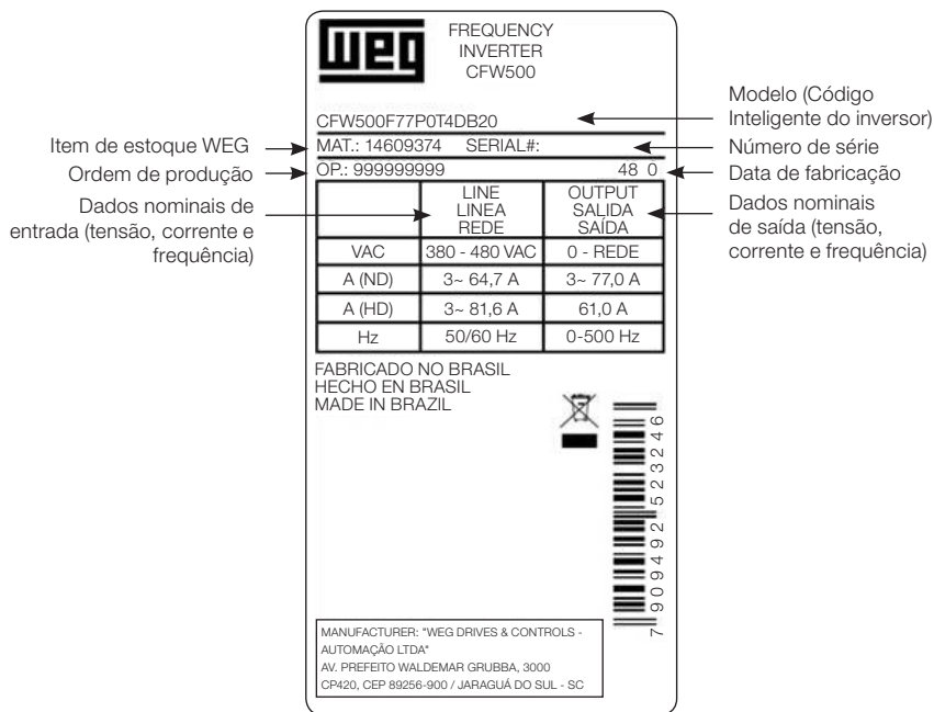
b) Etiqueta lateral do CFW500 para a mecânica F
