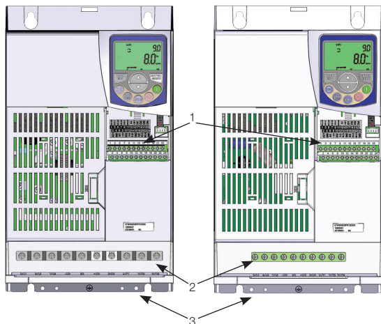
Frame Size D (200 V line) Tamaño D (línea 200 V) Mecânica D (linha 200 V)
