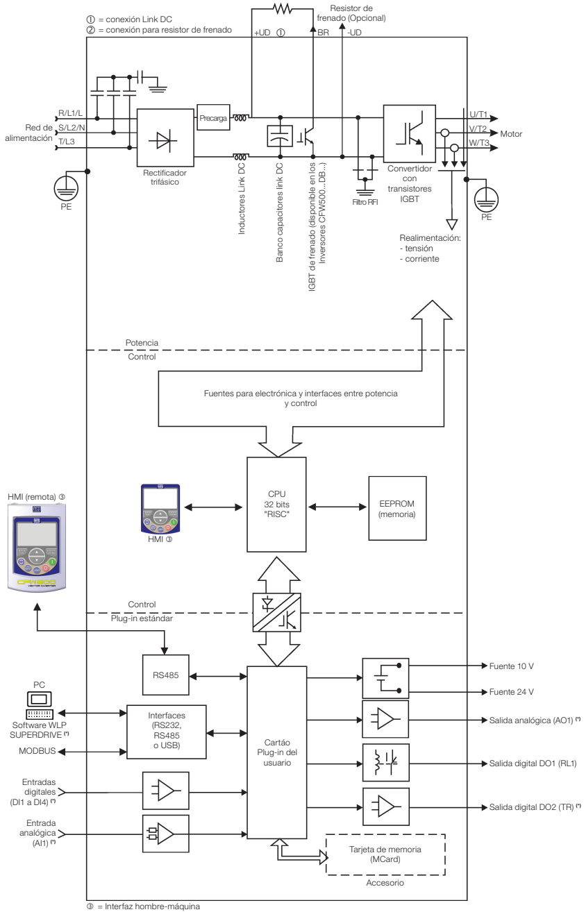
Figura 2.3: Diagrama de bloques del CFW500 para los tamaño F
