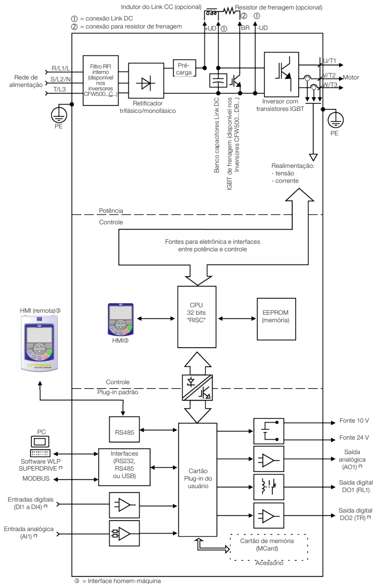
Figura 2.2: Blocodiagrama da CFW500 para mecânicas D e E
