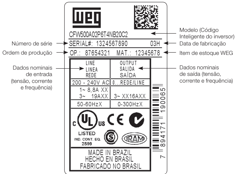
a) Etiqueta lateral do CFW500 para as mecânicas A a E
