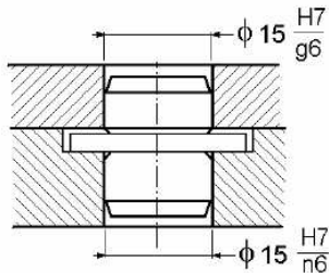
cavilha de centragem
