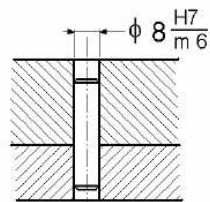
Referência com cunha cilíndrica
