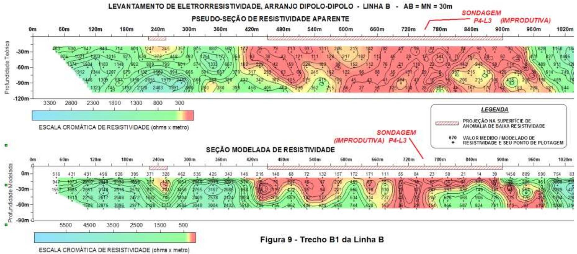
Figura 9 – Trecho B1 da pseudo-seção e seção modelada de resistividade da Linha B Figure 9 - Part B1 of pseudo-section and modeled section of resistivity of Line B
