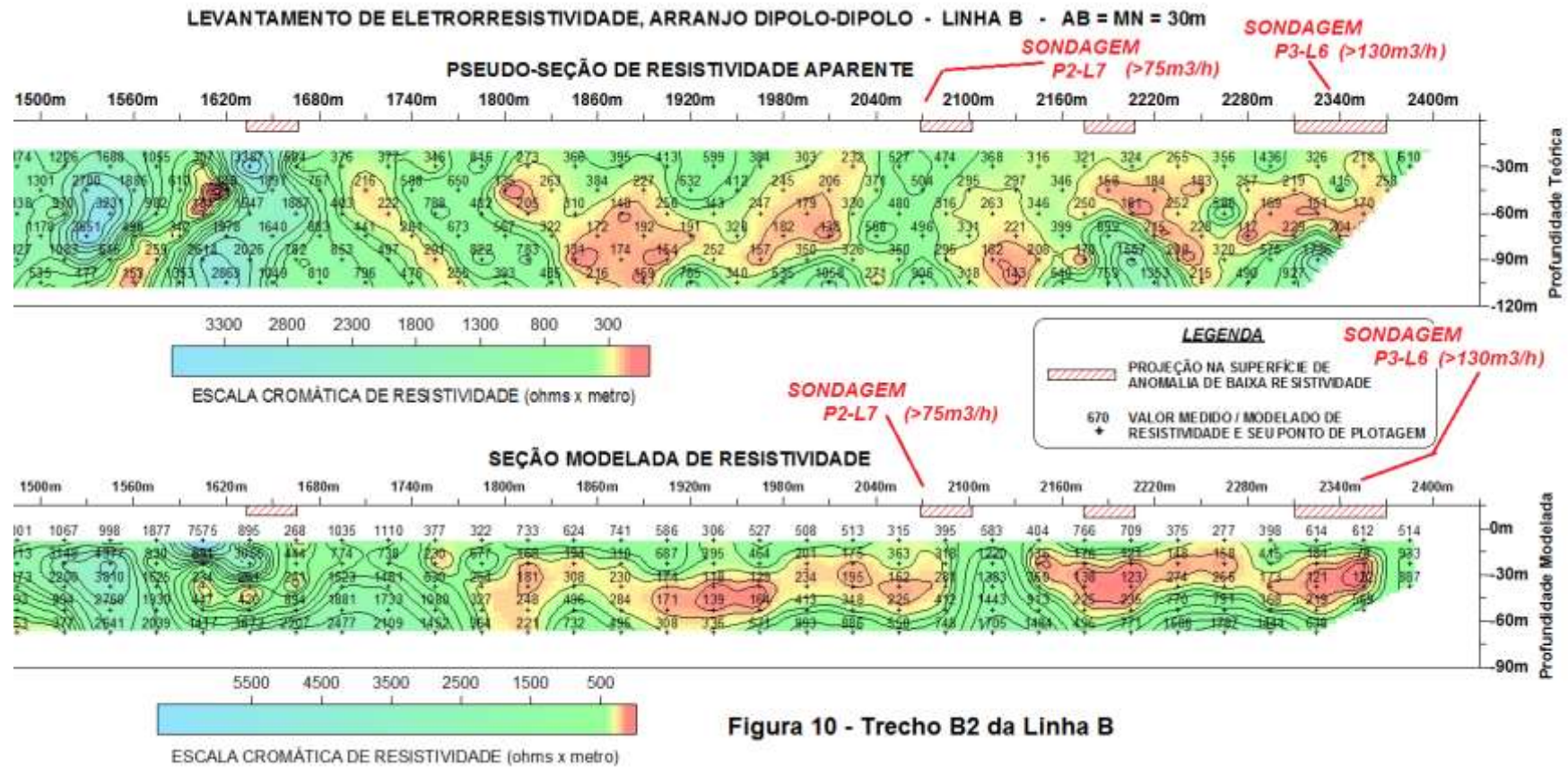
Figura 10 – Trecho B2 da pseudo-seção e seção modelada de resistividade da Linha B Figure 10 - Part B2 of pseudo-section and modeled section of resistivity of Line B
