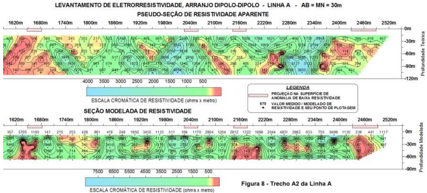
Figura 8 – Trecho A2 da pseudo-seção e seção modelada de resistividade da Linha A Figure 8 - Part A2 of pseudo-section and modeled section of resistivity of Line A
