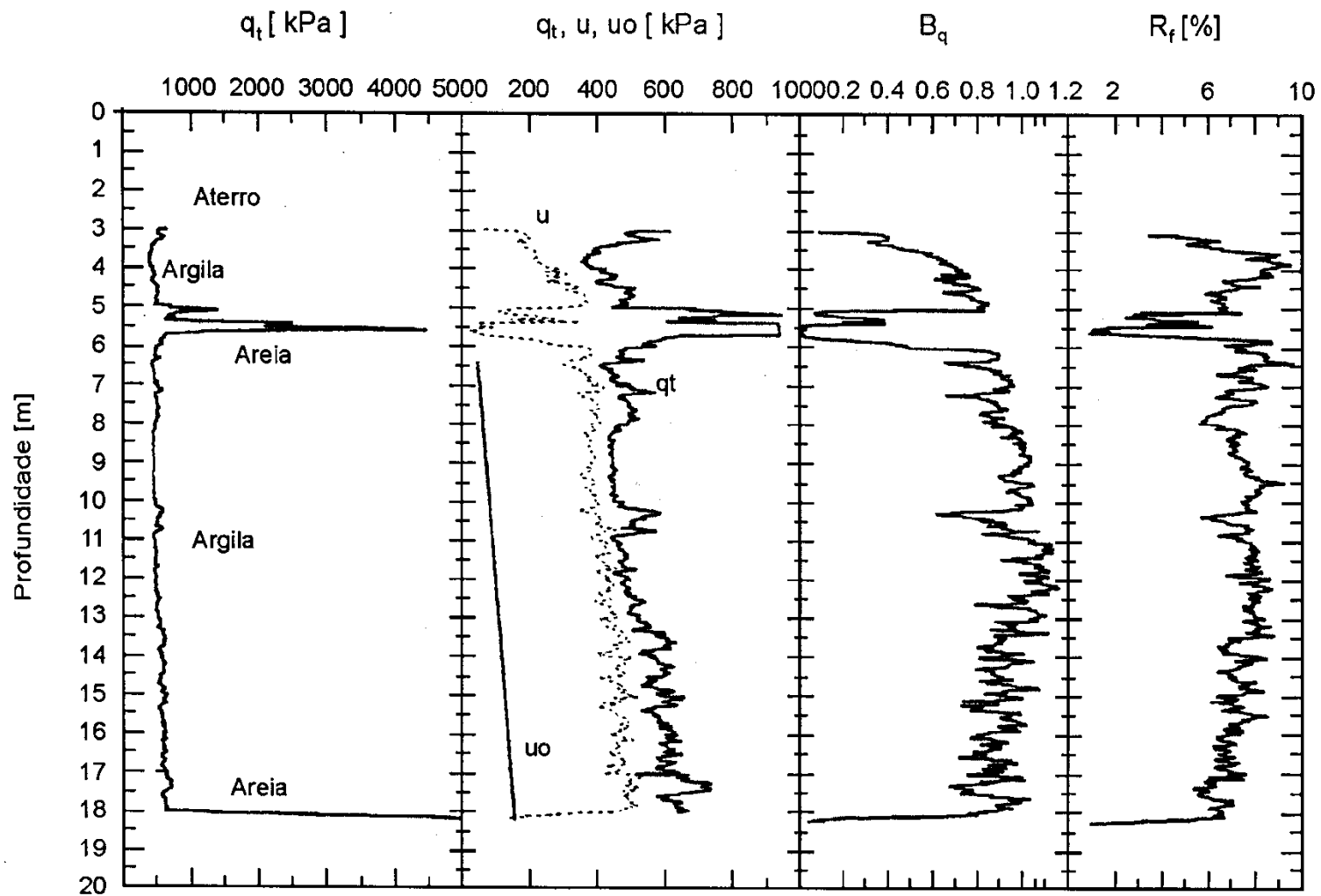
Resultado de um ensaio de piezocone na BR101 em Santa Catarina (Schnaid, 2000).
