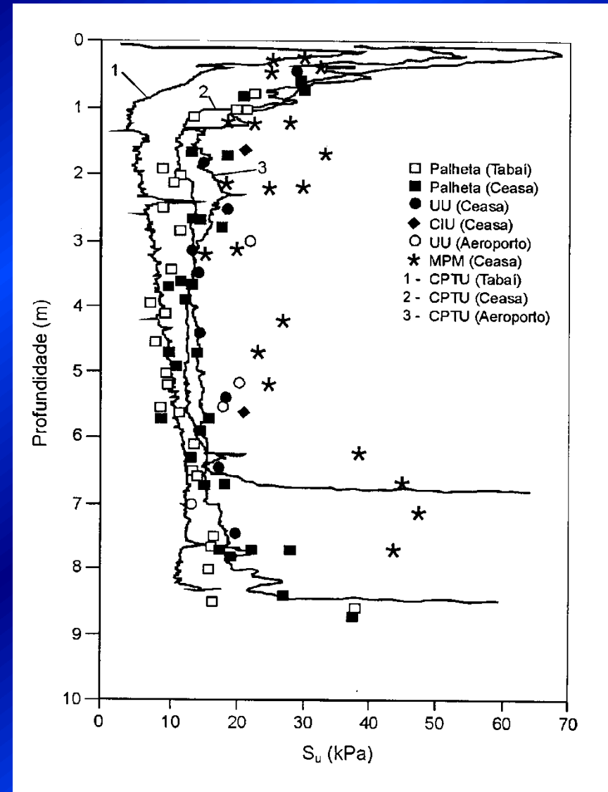
Varição de S_u com a profundidade (Schnaid, 2000).
