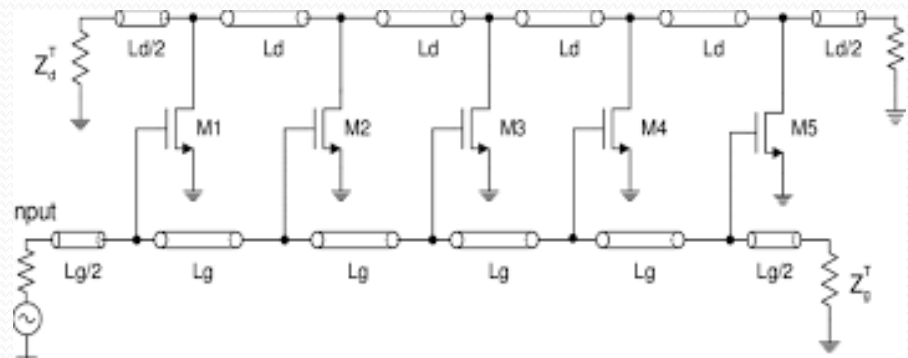
Amplificador distribuído usando linhas de transmissão
