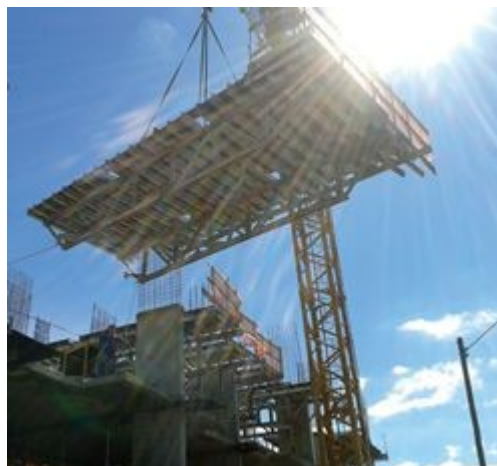
Economia de mão de obra e redução do cronograma são as principais vantagens trazidas pelas mesas voadoras, solução que une fôrma e escoramento em um mesmo sistema
