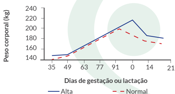
Gráfico 1 - Peso corporal de porcas alimentadas com diferentes níveis energéticos na gestação. Dia 0 é o dia do parto.
