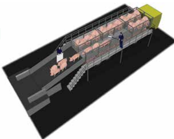
Figura 3 – Desembarque com a retirada dos suínos por compartimentos e utilização de auxílios de manejo adequados
