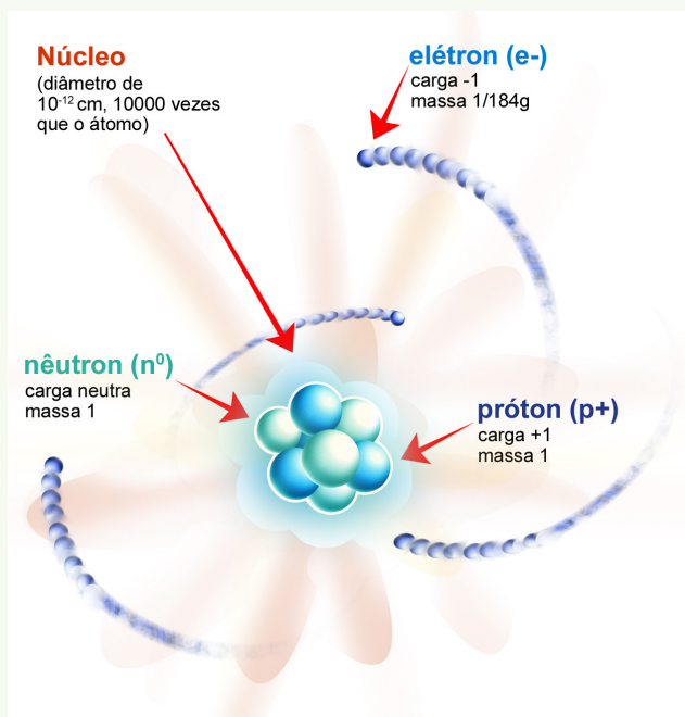
Figura 11.9: O átomo e seus constituintes
