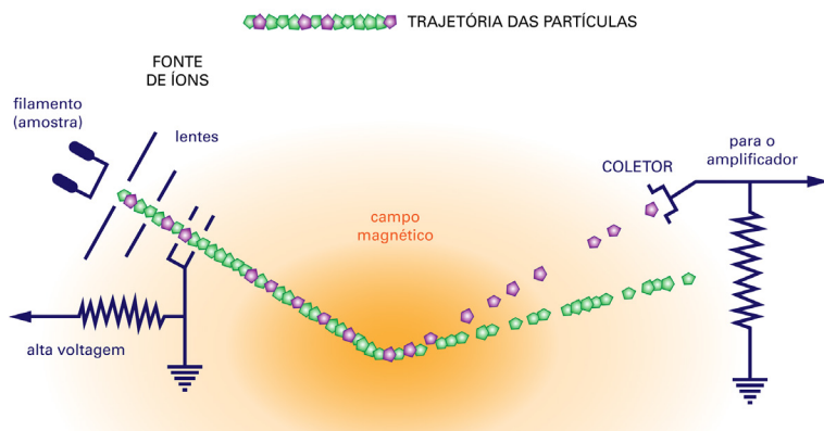
Figura 11.8: Esquema simplificado dos componentes de um espectrômetro de massa.
