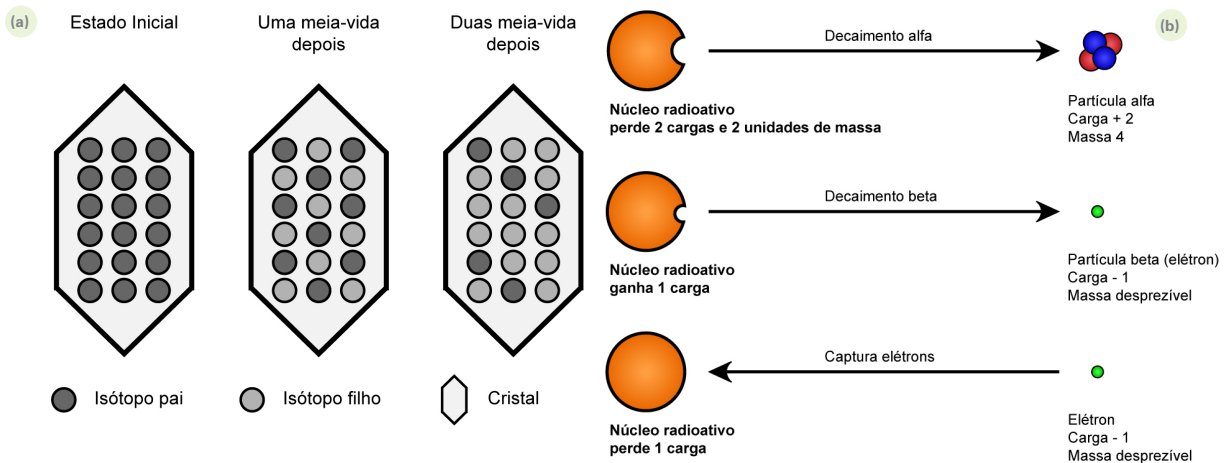
Figura 11.10: a) Conceito de meia-vida para um isótopo radioativo. Por definição, corresponde ao tempo necessário para que a metade dos átomos originais do elemento-pai (radioativo) se transforme em átomos estáveis do elemento-filho (radiogênico). Por exemplo, decorrido o tempo equivalente a uma meia-vida, a metade de 1.000 átomos de um elemento radioativo se transformará em 500 átomos estáveis (radiogênicos), restando ainda 500 átomos instáveis (radioativos). Após duas meias-vidas haverá 750 átomos estáveis e apenas 250 átomos instáveis, e assim por diante; b) Os três tipos de decaimento radioativo que ocorrem naturalmente em minerais. No decaimento alfa (a) ocorre a perda, pelo núcleo do átomo radiogênico, de dois prótons e dois nêutrons; o número de massa diminui de quatro e o número atômico, de dois. Na desintegração beta, o núcleo do átomo radiogênico emite um elétron de alta velocidade; um de seus nêutrons se transforma em um próton e o número atômico aumenta de um. Na captura de elétrons, um próton do núcleo captura um elétron orbital e se transforma em um nêutron; o número atômico diminui de um. A desintegração beta e a captura de elétrons não mudam o número de massa do elemento.
