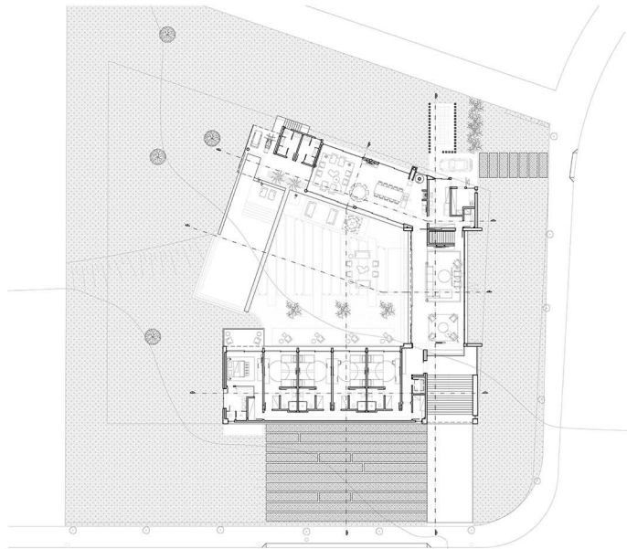
PLANTA TÉRREO
