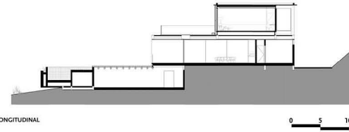
CORTE LONGITUDINAL
