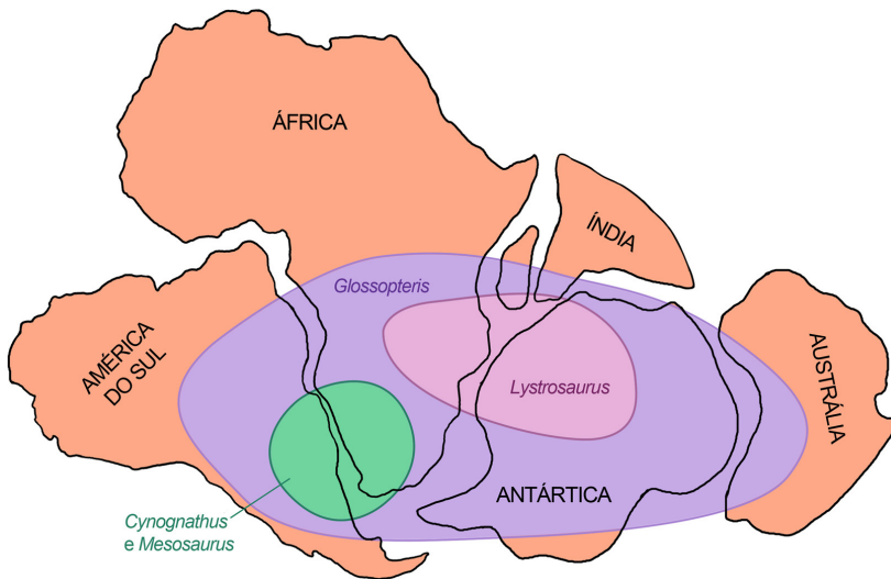
Figura 4.5: Distribuição de fósseis assemelhados, que corrobora a existência do supercontinente Pangeia: A. Répteis Lystrosaurus (África, Índia, América do Sul) e Mesosaurus (África e América do Sul); B. Fauna Glossopteris (ocorrência em todos os continentes meridionais e na Índia).
