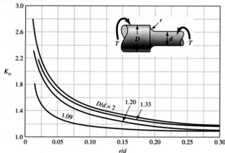
Figura 11- Fator de concentração de tensão ( k_t ) para eixo de seção circular sujeito a torção
