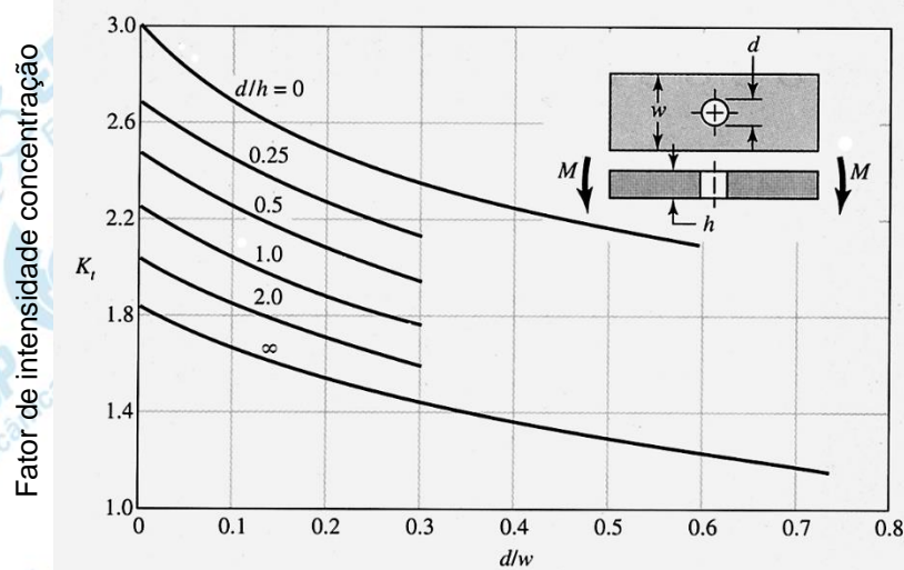
Figura 5- Fator de concentração de tensão ( k_t ) para uma barra retangular sujeita à flexão com um furo transversal
