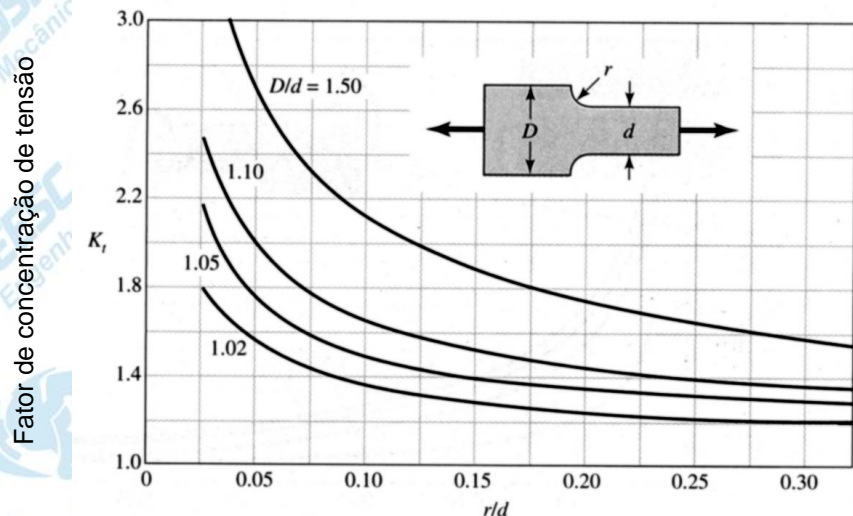
Figura 8- Fator de concentração de tensão ( k_t ) para uma barra com variação de secção sujeita a tração e compressão.
