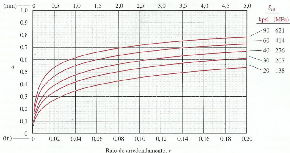
Fatores de sensibilidade ao entalhe para alumínio tratado termicamente (-T)
