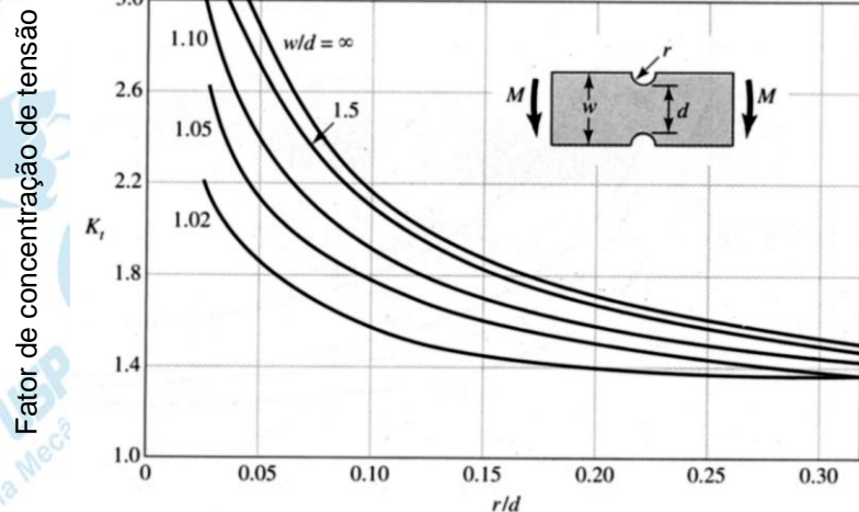
Figura 7- Fator de concentração de tensão ( k_t ) para uma barra retangular sujeita à flexão
