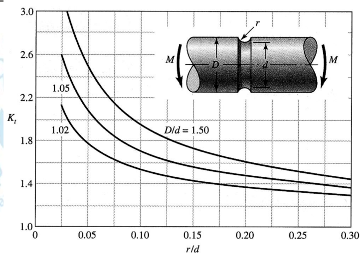
Figura 17- Fator de concentração de tensão ( k_t ) para eixo de seção circular, com rasgo arredondado, sujeito à flexão.
