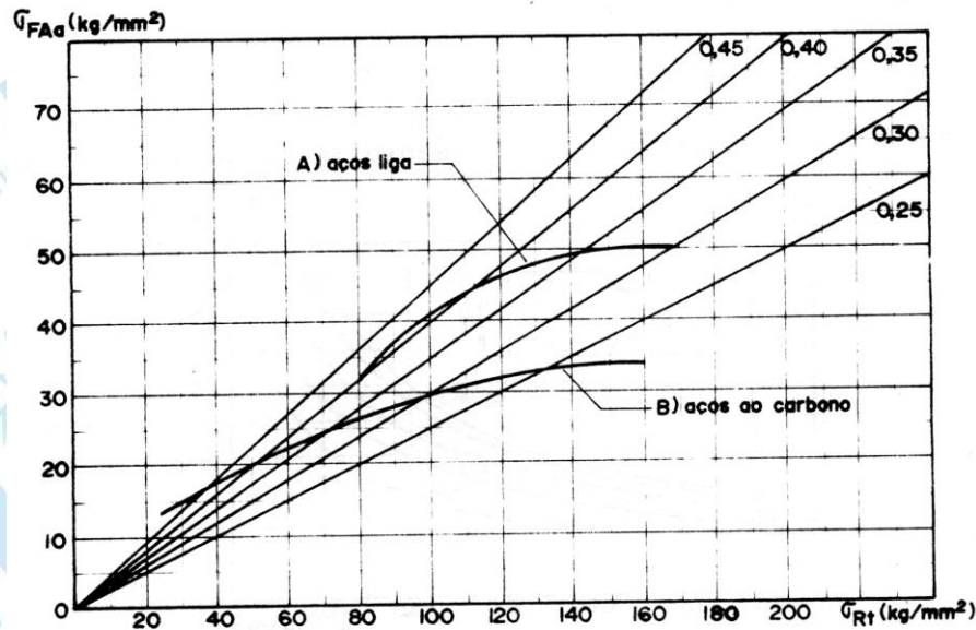
Figura 2- Curvas do limite de resistência à fadiga alternada AXIAL para aços em função da tensão de ruptura a Tração. (para axial pura)
