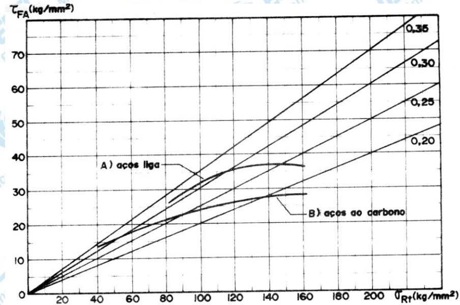
Figura 3- Curva do limite de resistência à fadiga alternada de TORÇÃO para aços em função da tensão de ruptura a Tração. (para torção pura)
