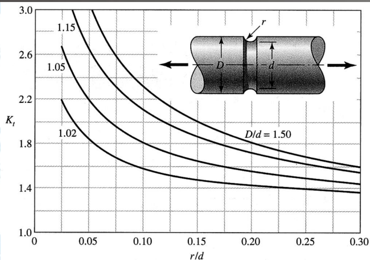
Figura 16- Fator de concentração de tensão ( k_t ) para eixo de seção circular, com um rasgo arredondado, sujeito à tração.
