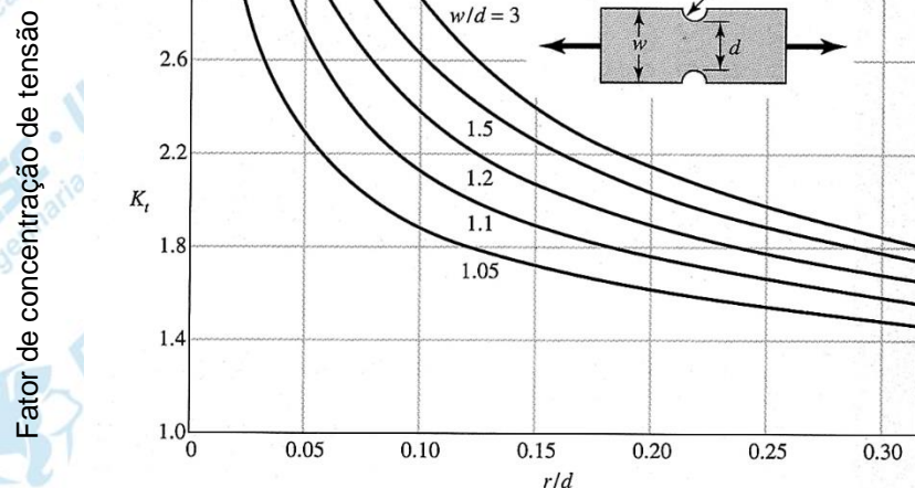
Figura 6- Fator de concentração de tensão ( k_t ) para uma barra com entalhes, sujeita a tração e compressão
