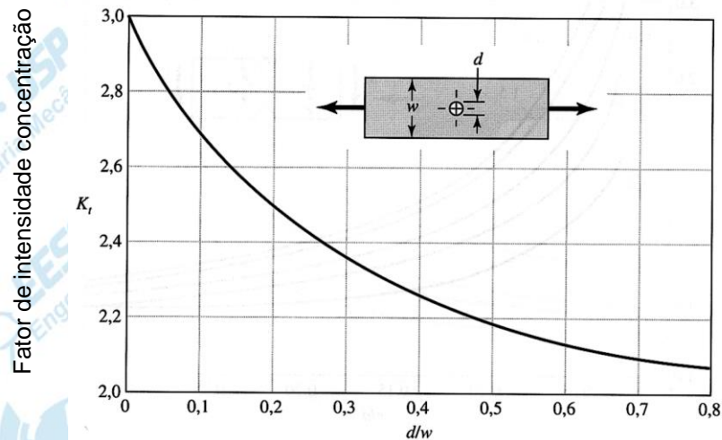
Figura 4- Fator de concentração de tensão ( k_t ) para uma barra retangular sujeita à tração ou compressão com um furo transversal
