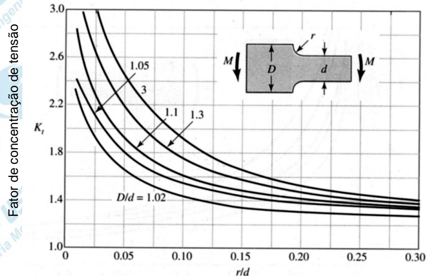
Figura 9- Fator de concentração de tensão ( k_t ) para uma barra com variação de secção sujeita a flexão.
