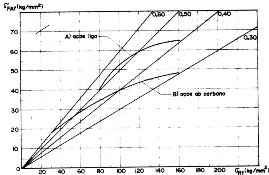
Figura 1- Curvas do limite de resistência à fadiga alternada de FLEXÃO para aços em função da tensão de ruptura a tração (para flexão pura e mista).
