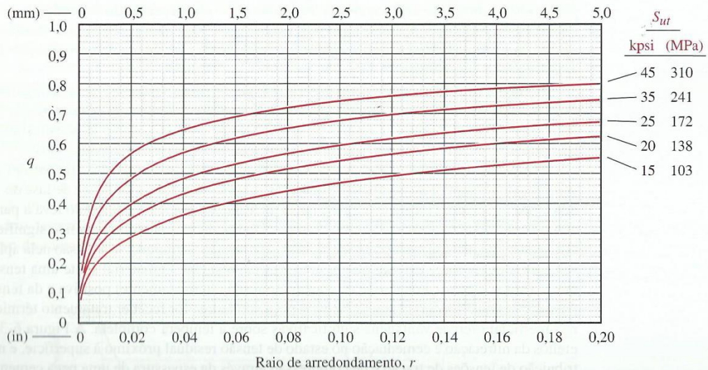
Fatores de sensibilidade ao entalhe para alumínio recozido e encruado (-O e -H)
