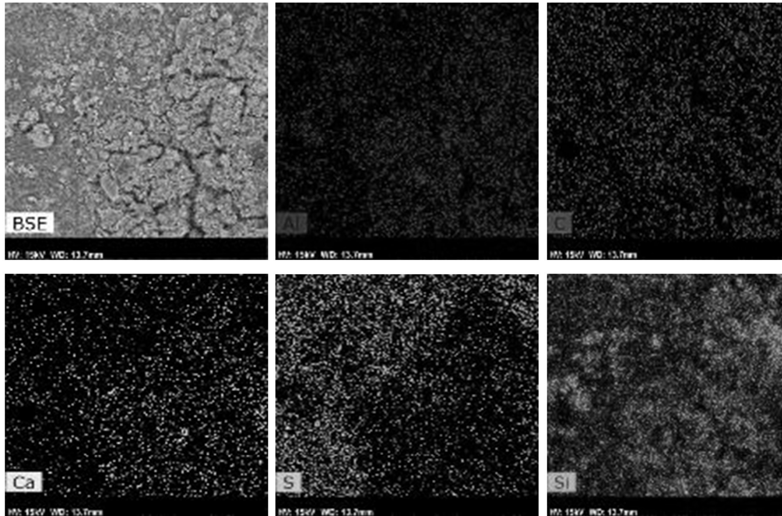
Micrografia de uma membrana com depósitos e resultados da análise de caracterização dos depósitos por EDX
