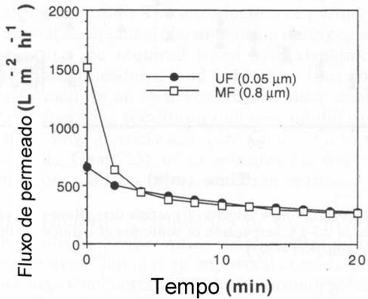
Efeito da formação de torta em membranas de MF e UF
