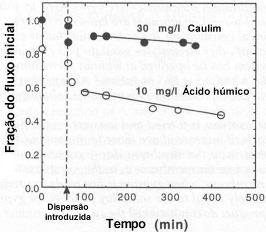
Efeitos das substâncias orgânicas no fluxo de permeado
