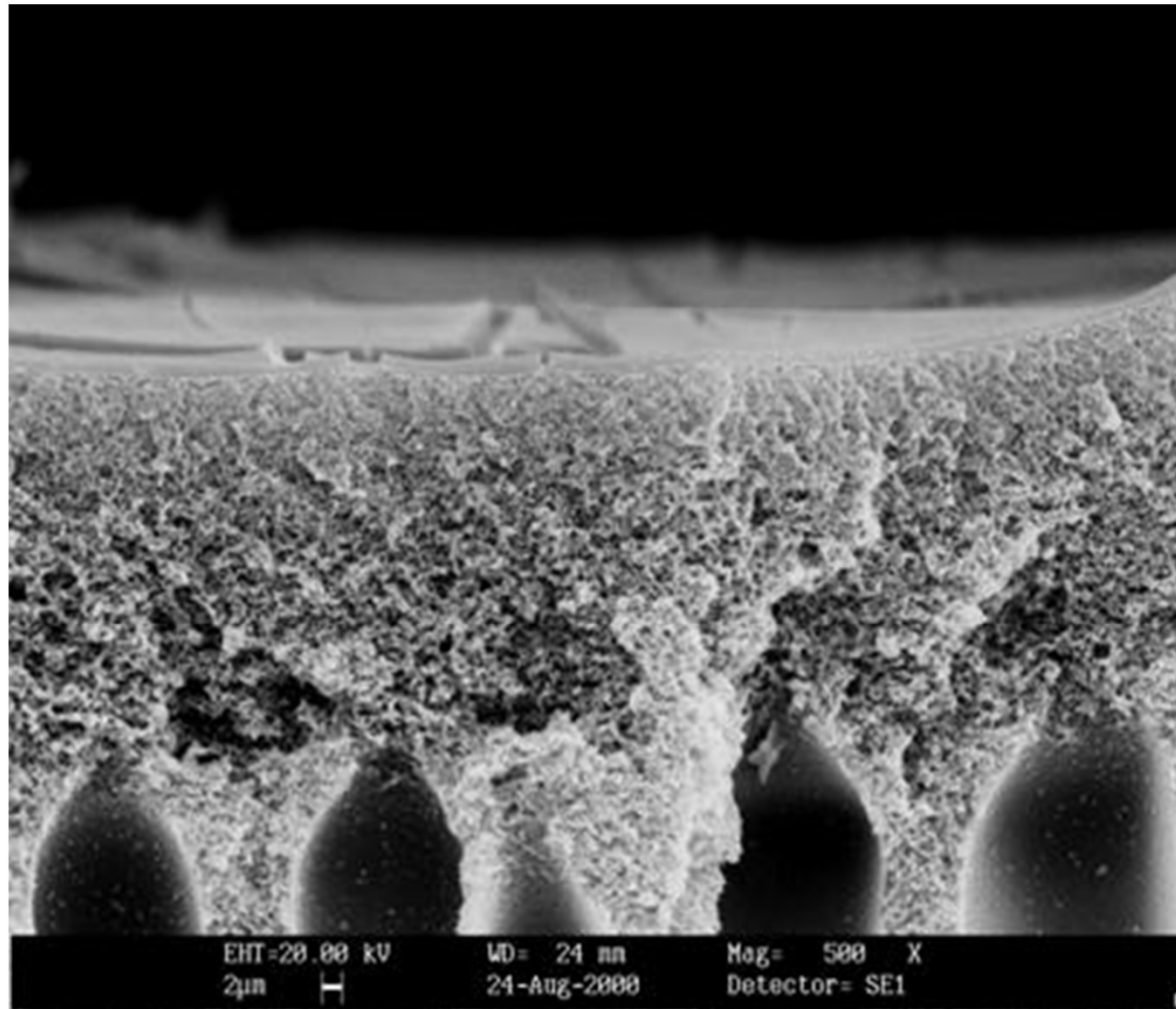
Formação de depósito orgânico sobre uma membrana de UF
