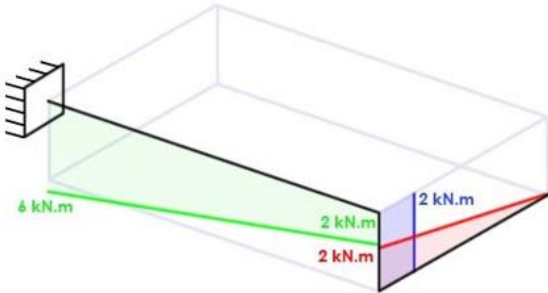
MOMENTO FLETOR
