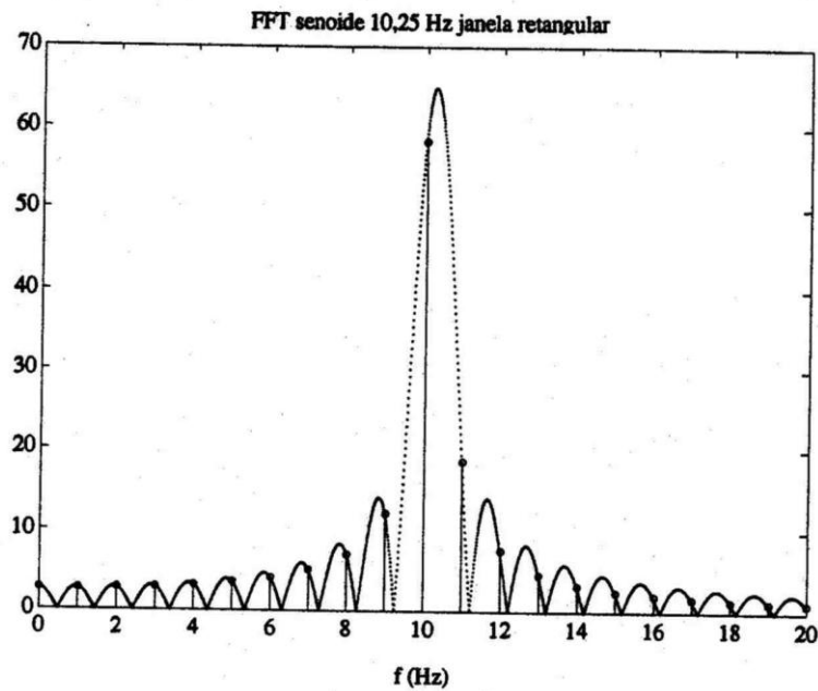
Figura 2 - Módulo do espectro da TDF de cossenóide de 10,25 Hz, truncada por janela retangular e amostrada.
