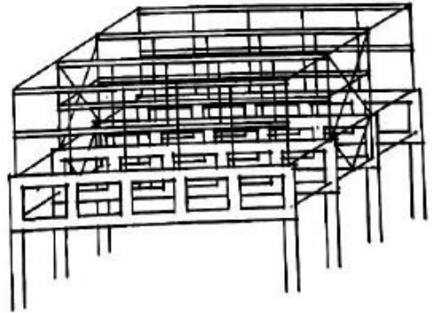
Geschoßbrücken-Systeme Storey bridge systems
