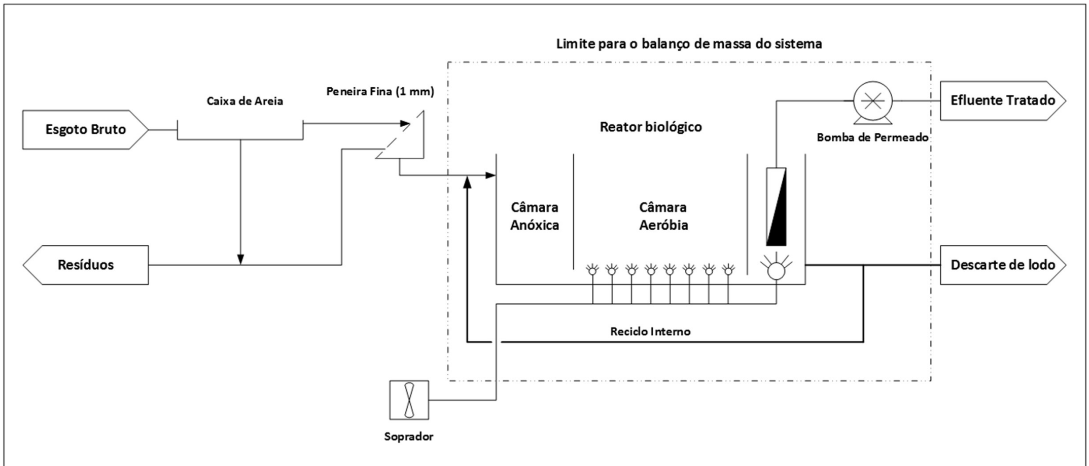
Sistema para remoção de matéria orgânica e de nitrogênio
