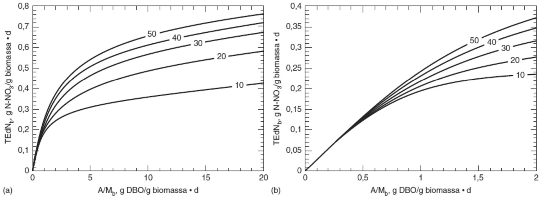
FIGURA 8-31 Taxas específicas de desnitrificação (TEdN b ), com base na concentração de biomassa, a 20°C, em função da relação alimento/microrganismos (A/M b ), para várias porcentagens de DQOrb em relação à DQOb do afluente (a) para valores de A/M b até 20 e (b) escala expandida para valores de A/M b até 2.
