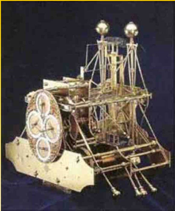
Cronômetro marítimo H1 de Harrison (1730)
