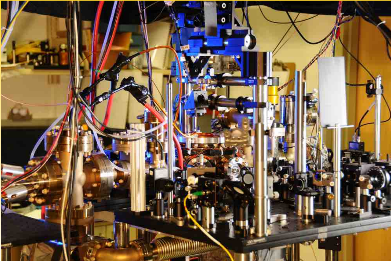
Relógio atômico de Ytérbio do NIST, com precisão de 10^{-18} s
