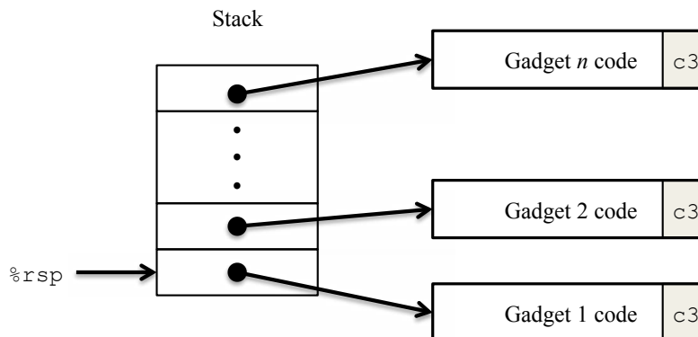
Figura 2: Preparando uma sequência de gadgets para execução. O valor 0xc3 codifica a instrução ret .
