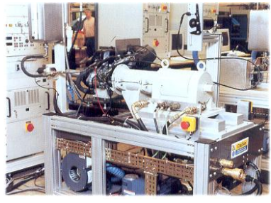
dinamômetro
